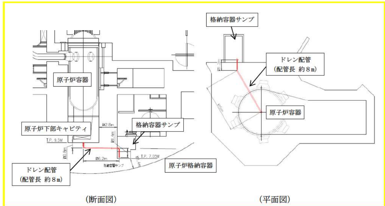
図2 格納容器サンプの配置及びドレン配管形状
