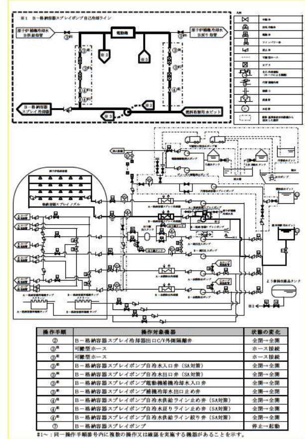
第1.6.15図 B-格納容器スプレイポンプ（自己冷却）による原子炉格納容器内へのスプレイ（炉心損傷後） 概要図
