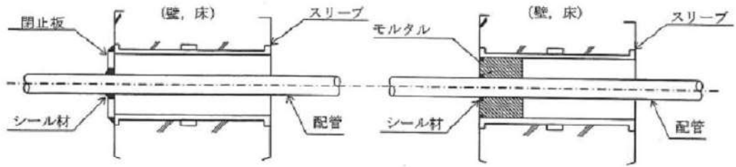
(a) 閉止板等による漏えい防止図 (床面部, 壁面部)
