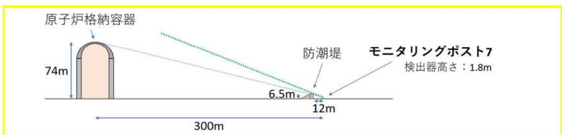
第2図 モニタリングポスト7から3号炉の原子炉方向を見たときの新設防潮堤との位置関係
