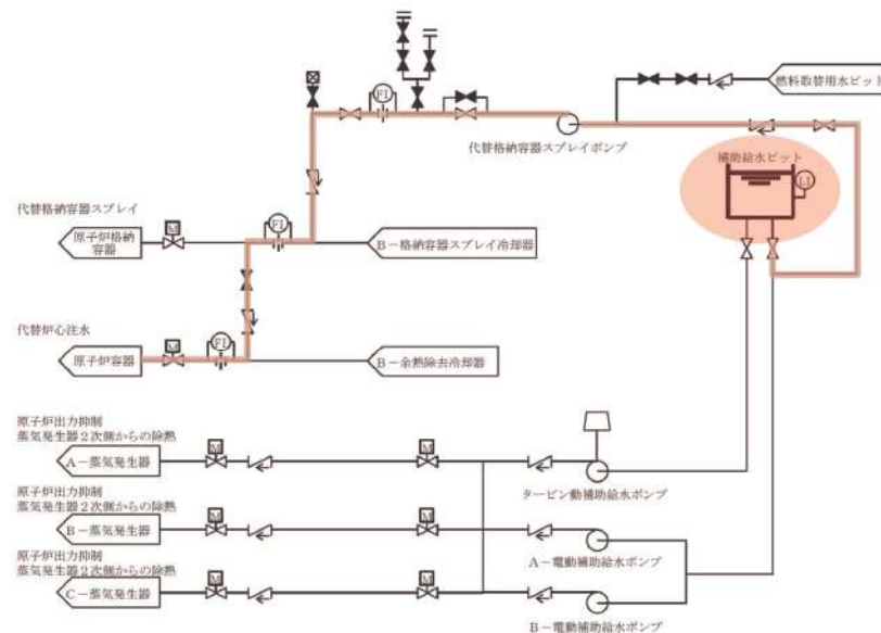
泊3号炉 重大事故等時に必要となる水源及び水の供給設備 系統概要図
