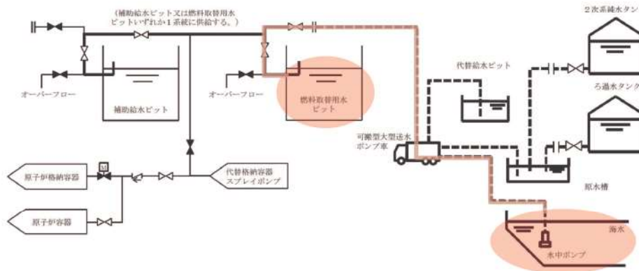
泊3号炉 重大事故時に必要となる水源及び水の供給設備 系統概要図
