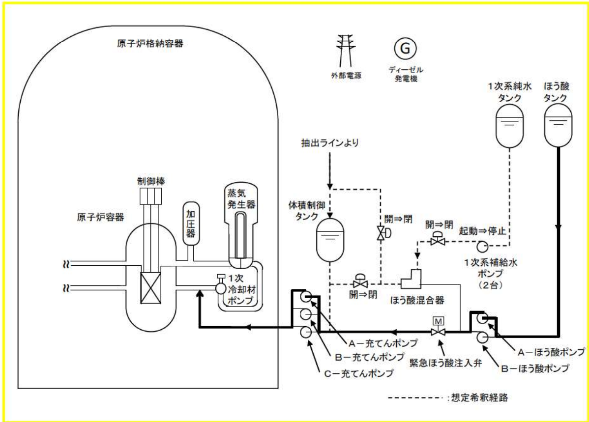
第7.4.4.1図 「反応度の誤投入」の重大事故等対策の概略系統図 (ほう酸注入)
