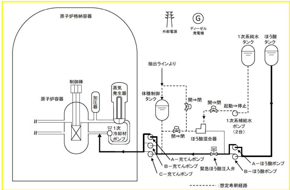
図1 「原子炉起動時に、化学体積制御系の弁の誤動作等により原子炉へ純水が流入する事故」の重大事故等対策の概略系統図 (ほう酸注入)
