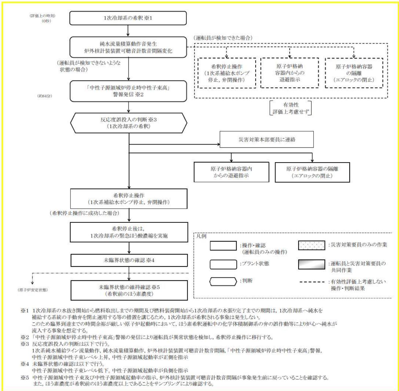
第7.4.4.2図 「反応度の誤投入」の対応手順の概要 (「原子炉起動時に、化学体積制御系の弁の誤動作等により原子炉へ純水が流入する事故」の事象進展)
