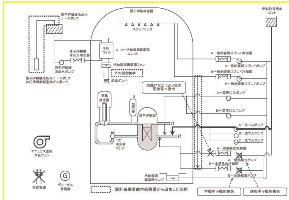
図1 「燃料取出前のミッドループ運転中に原子炉冷却材圧力バウンダリが喪失する事故」の重大事故等対策の概略系統図 (炉心注水)
