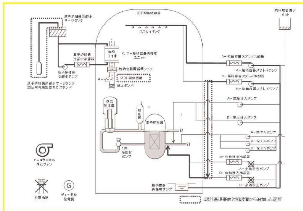
図2 「燃料取出前のミッドループ運転中に原子炉冷却材圧力バウンダリが喪失する事故」の重大事故等対策の概略系統図 (代替再循環、格納容器スプレイ再循環及び格納容器内自然対流冷却)
