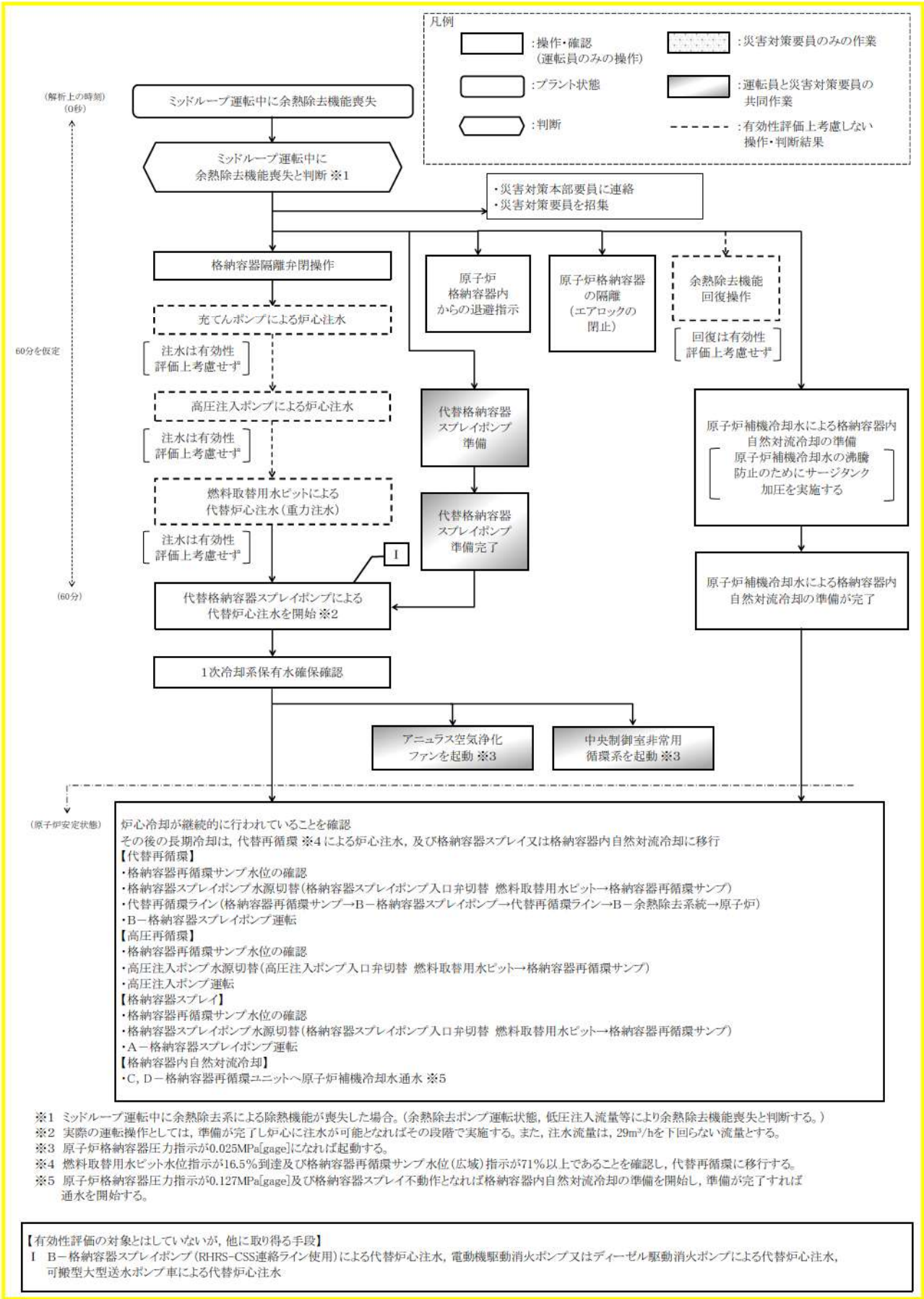
第 7. 4. 1. 2 図 「崩壊熱除去機能喪失 (余熱除去系の故障による停止時冷却機能喪失)」 の対応手順の概要 (「燃料取出前のミッドループ運転中に余熱除去機能が喪失する事故」の事象進展)
