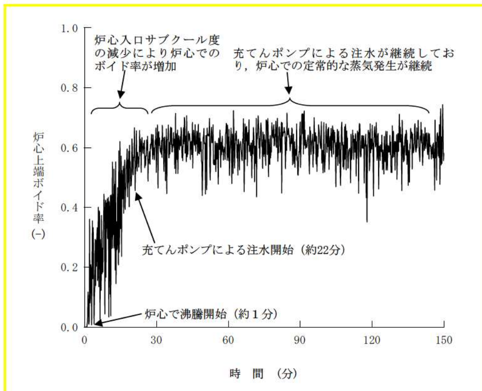
図4 原子炉冷却材の流出時の炉心上端ボイド率の推移
