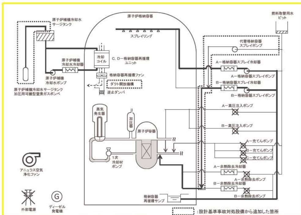
図2 「燃料取出前のミッドループ運転中に余熱除去機能が喪失する事故」の重大事故等対策の概略系統図 (代替再循環, 格納容器スプレイ再循環及び格納容器内自然対流冷却)
