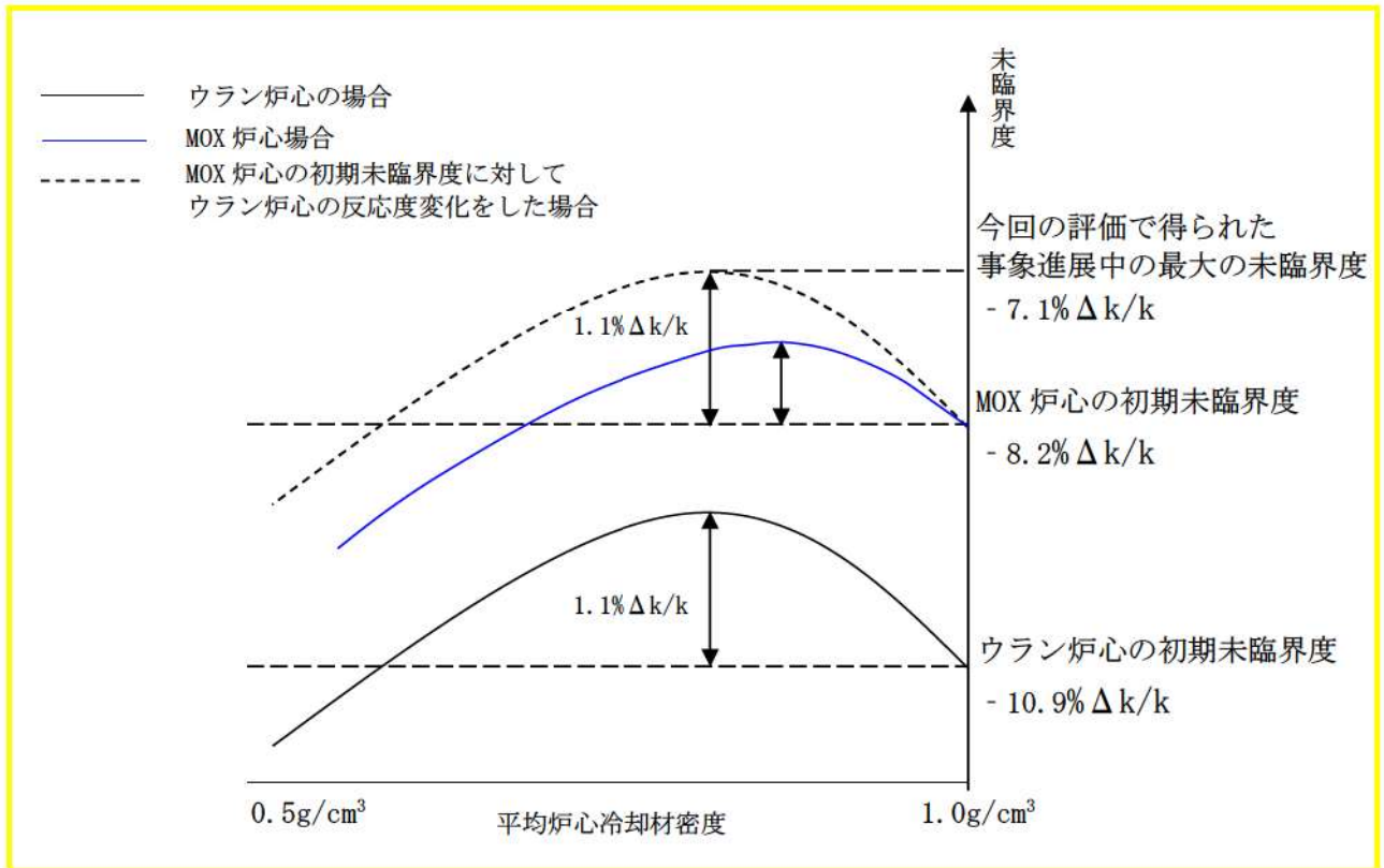
図6 ウラン炉心を利用した際の保守性についての概要図
