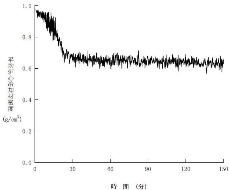
図3 原子炉冷却材の流出時の平均炉心冷却材密度の推移
