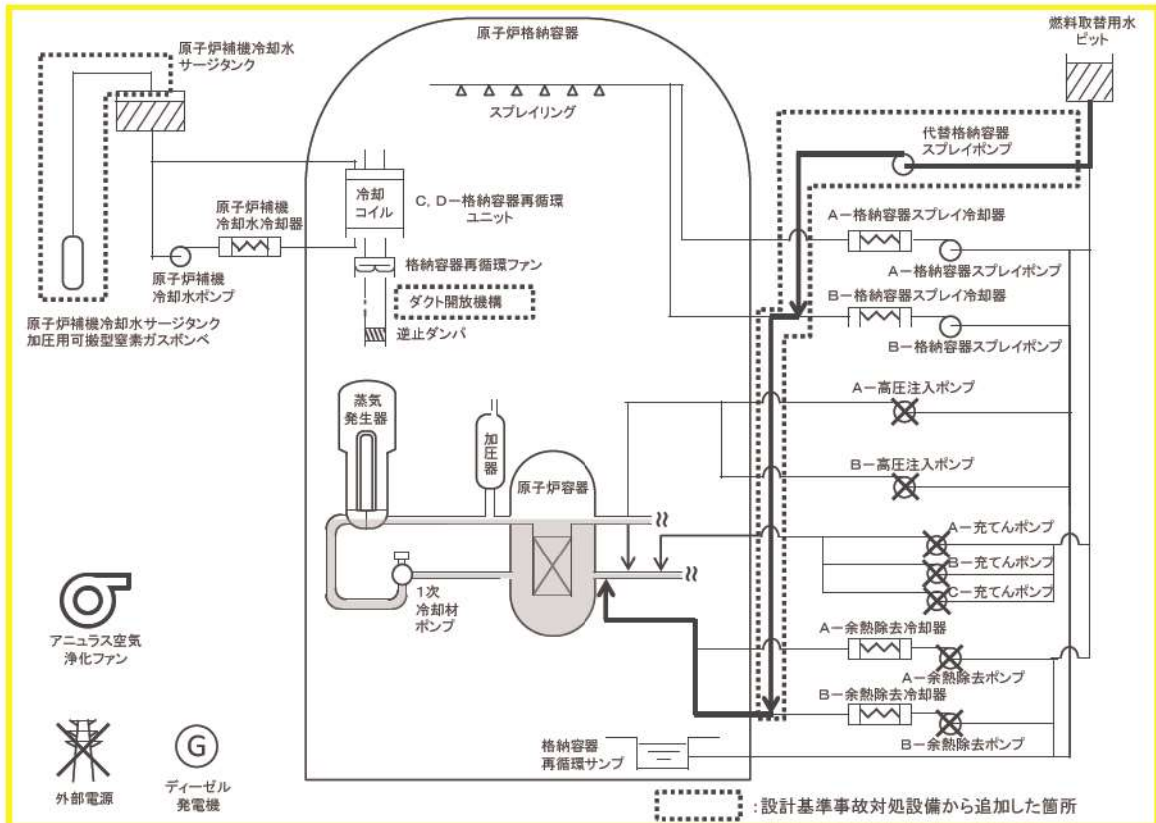
第7.4.1.1図 「崩壊熱除去機能喪失（余熱除去系の故障による停止時冷却機能喪失）」の重大事故等対策の概略系統図（1/2）（炉心注水）
