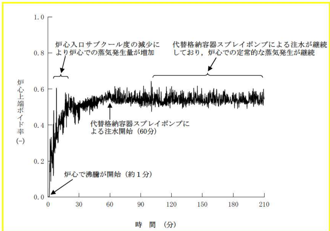
図2 崩壊熱除去機能喪失及び全交流動力電源喪失時の炉心上端ボイド率の推移
