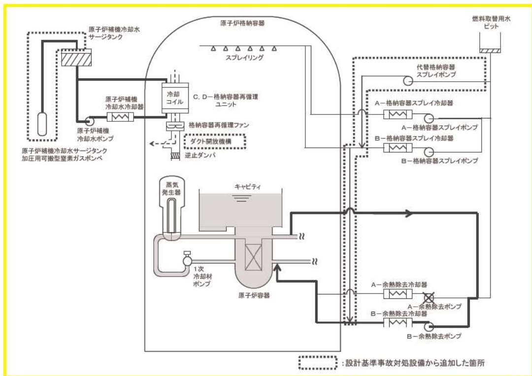
図1 重大事故対策概要図 (崩壊熱除去機能喪失、原子炉冷却材の流出の場合)
