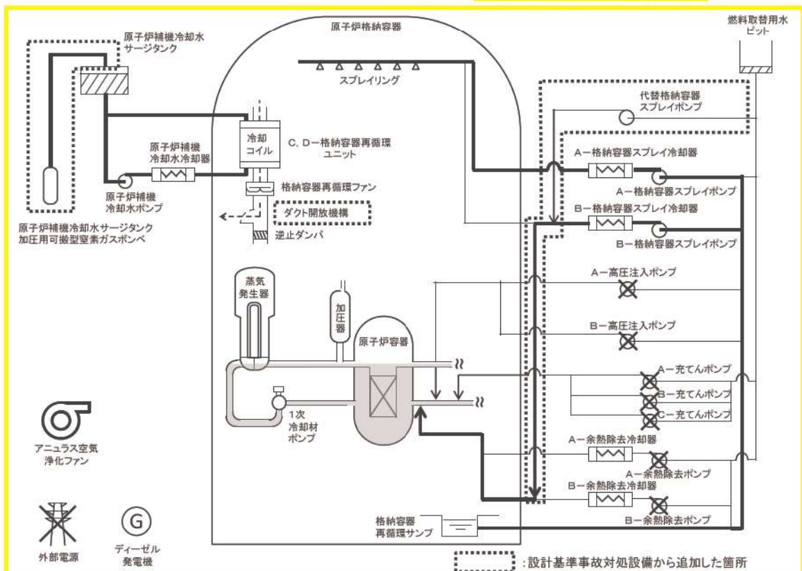
第7.4.1.1図 「崩壊熱除去機能喪失（余熱除去系の故障による停止時冷却機能喪失）」の重大事故等対策の概略系統図（2/2） （代替再循環、格納容器スプレィ再循環及び格納容器内自然対流冷却）
