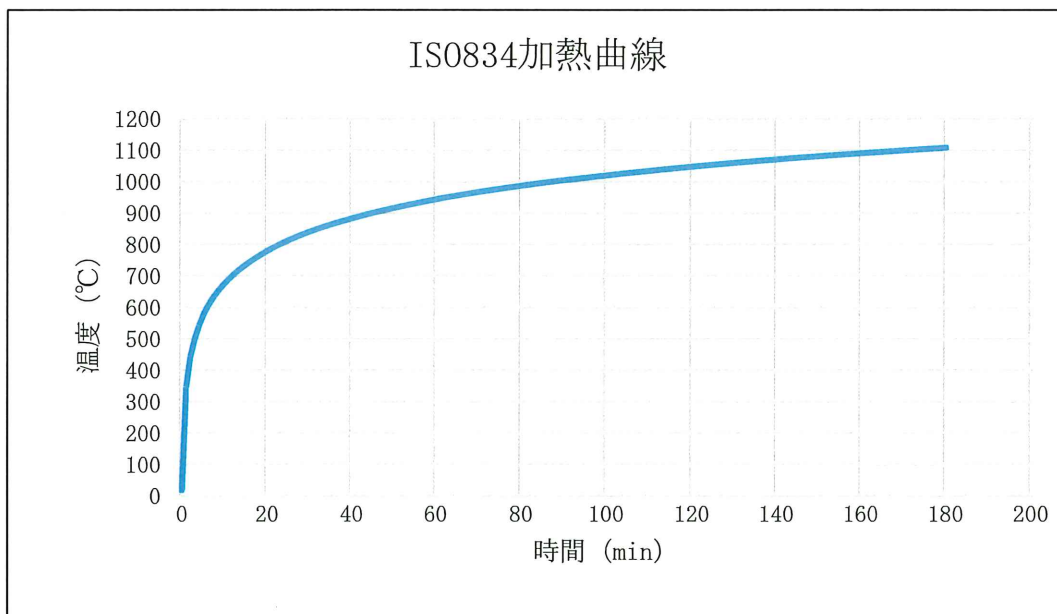
第6-1圖 加熱曲線
