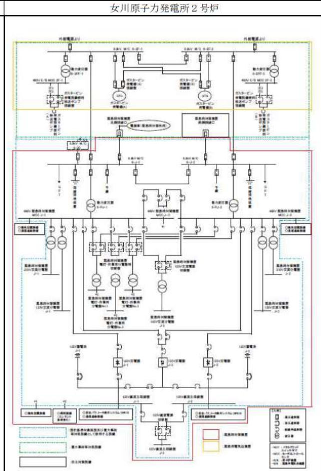
第 1.18-15 図 緊急時対策所 給電系統概要図
