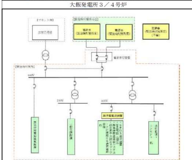
第 1.18.13 図 緊急時対策所 給電系統概要
