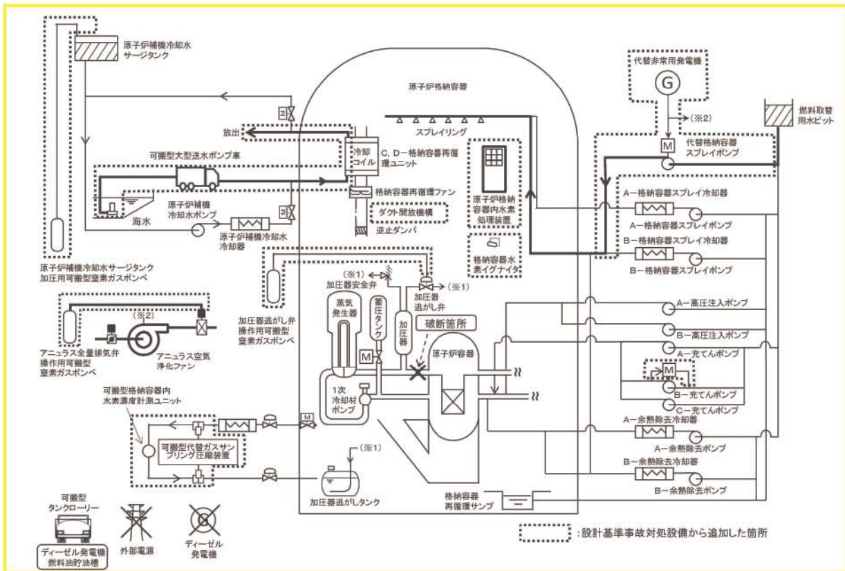
第 7.2.4.1 図 「水素燃焼」の重大事故等対策の概略系統図 (原子炉格納容器内水素処理装置及び格納容器水素イグナイタ)
