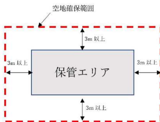
第 1-34 図：可搬型重大事故等対処設備の保管エリア
