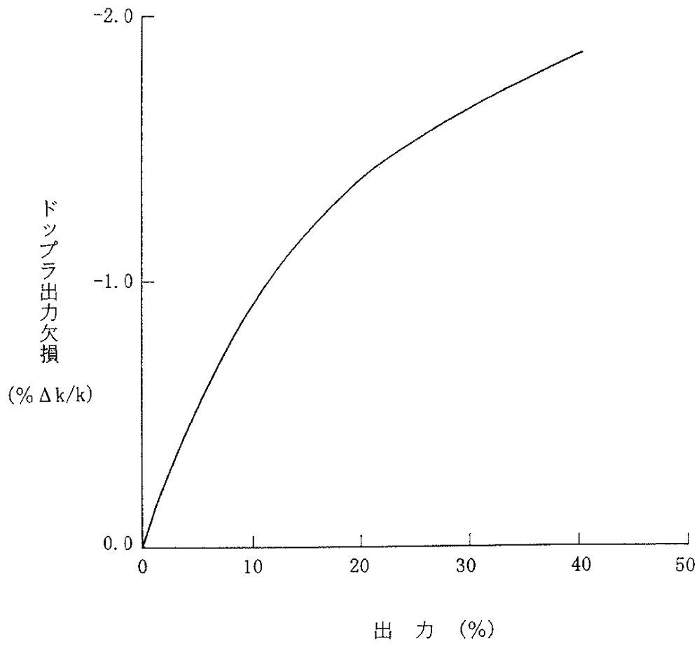
第1.5.3.2図 解析に使用したドップラ出力欠損
