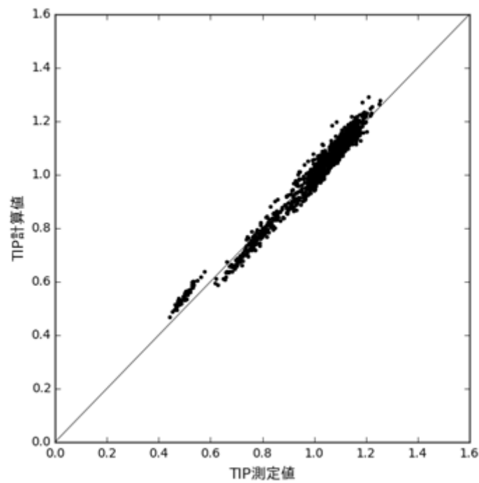
図 4.3-11 TIP 測定値と計算値の炉心平均軸方向分布の比較 (BWR 大型 C 格子炉の例)
