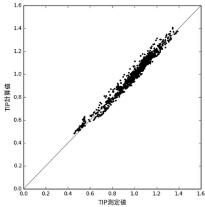
図 3-44 TIP 測定値と計算値の炉心平均軸方向分布の比較 (BWR 小型 S 格子炉の例)
