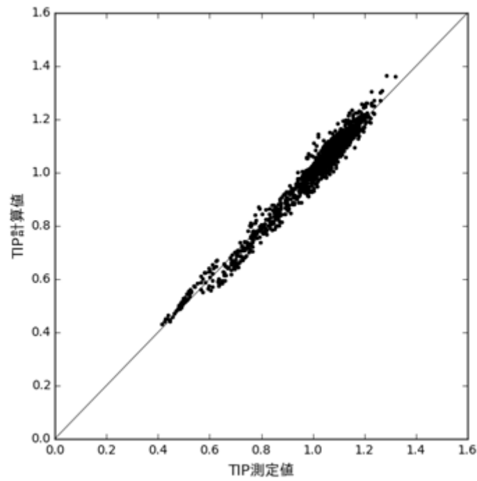
図 4.3-10 TIP 測定値と計算値の炉心平均軸方向分布の比較 (BWR 中型 S 格子炉の例)
