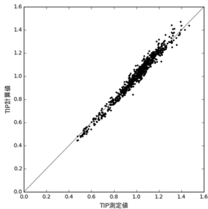
図 4.3-7 TIP 測定値と計算値の炉心平均軸方向分布の比較 (BWR 小型 D 格子炉の例)
