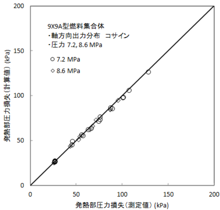
図 3-100 NUPEC 9 × 9 A 型燃料熱水力試験 発熱部圧力損失の比較 (二相試験)
