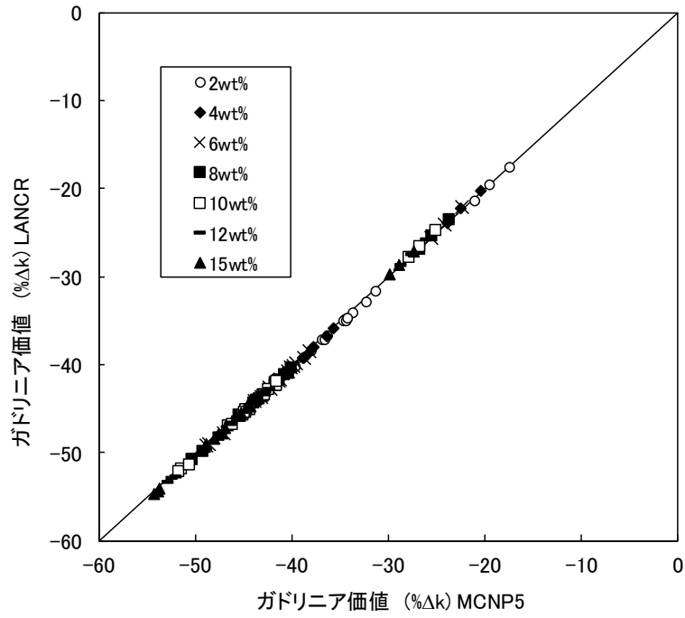
図 2-48 ガドリニア価値のモンテカルロ計算との比較
