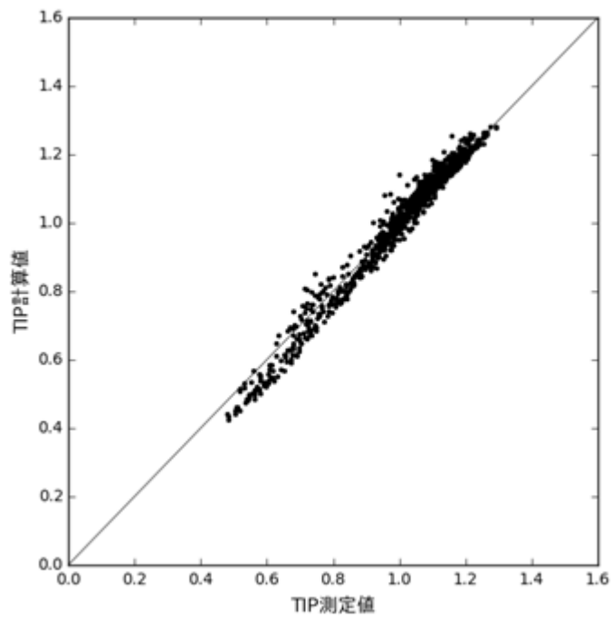
図 3-49 TIP 測定値と計算値の炉心平均軸方向分布の比較 (ABWR の例)
