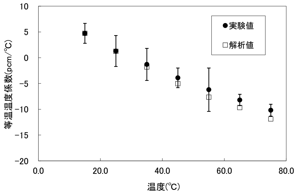
図 2-33 BASALA 臨界試験における等温温度係数の比較
