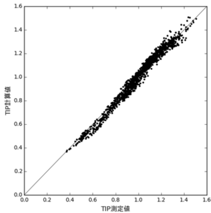
図 3-45 TIP 測定値と計算値の炉心平均軸方向分布の比較 (BWR 中型 D 格子炉の例)
