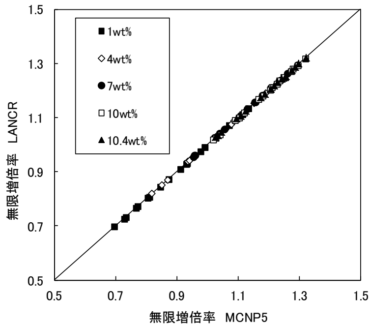
図 2-47 \text{PuF}_6 富化度ごとの無限増倍率のモンテカルロ計算との比較
