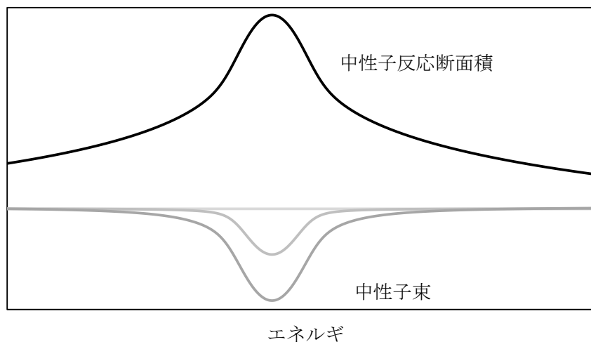
図 中性子反応断面積と中性子束
