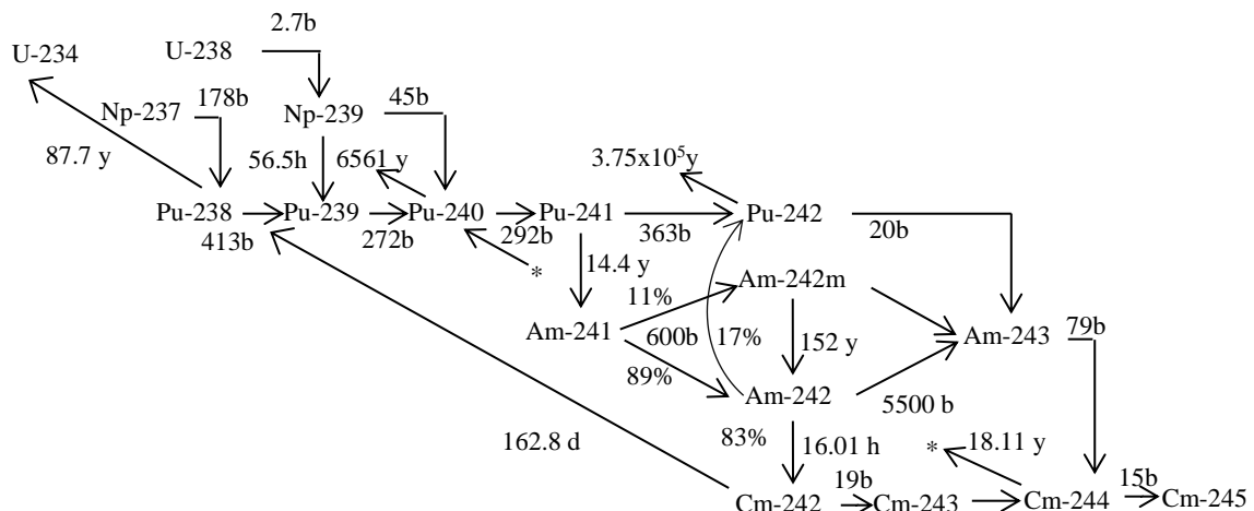
図 3.2-6 Pu-239 ~ Am-241 を含む崩壊系列 (2, 200m/sec 断面積)
