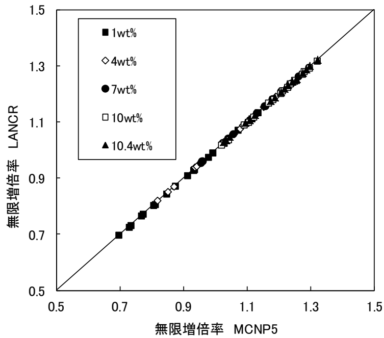
図 4.2-47 PuF 4 富化度ごとの無限増倍率のモンテカルロ計算との比較
