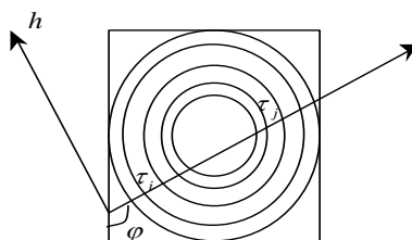
図 3.1-5 燃料ノード内の中性子パス
