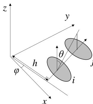
図 3.1-4 任意の二次元体系
