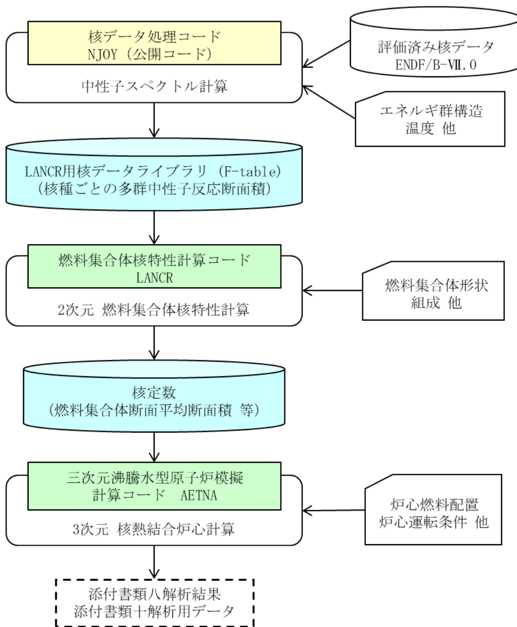
図 1.2-1 LANCR と AETNA を用いた炉心解析の流れ
