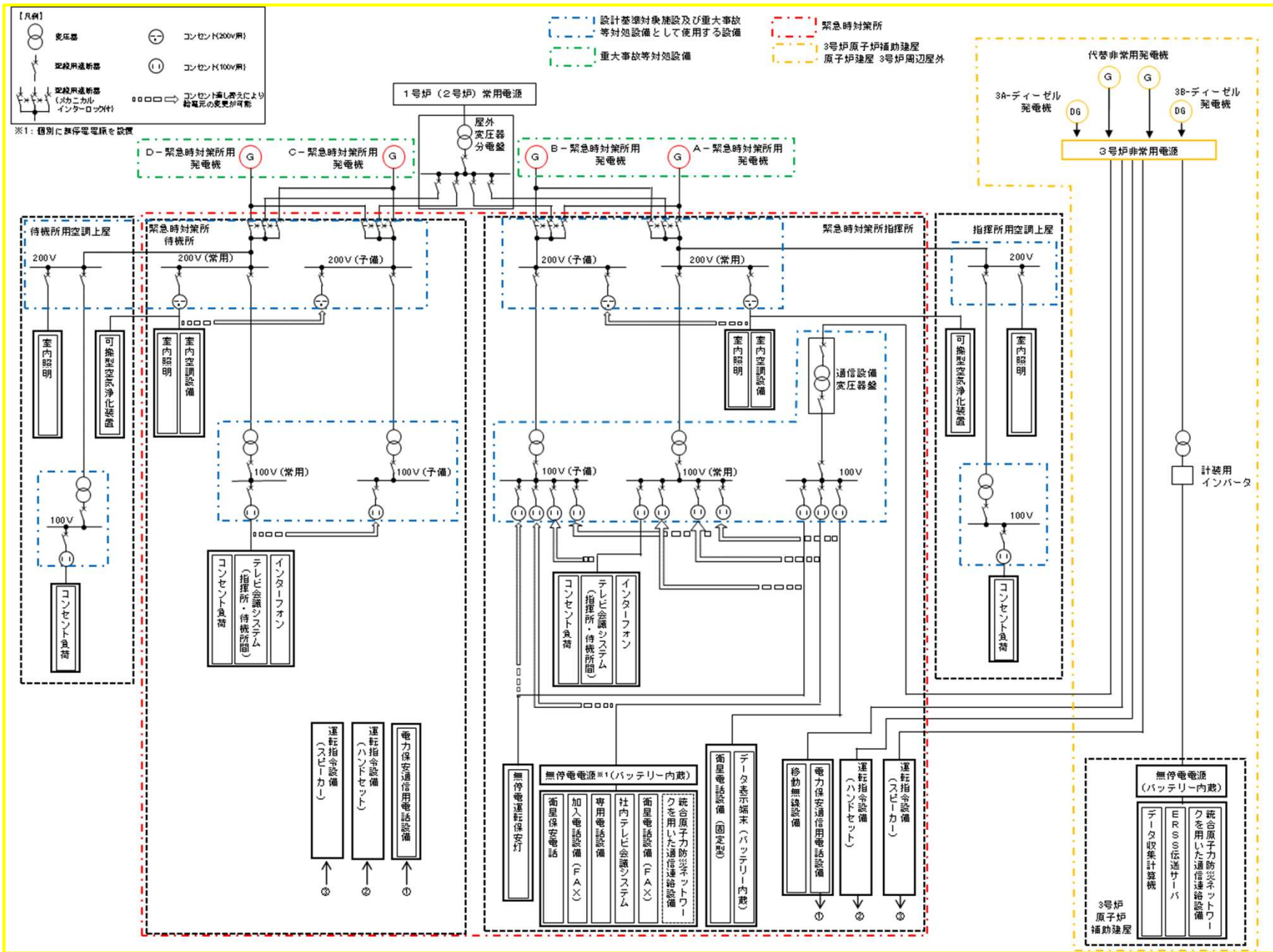
[61-14, (補足説明資料) 61-4系統図]
