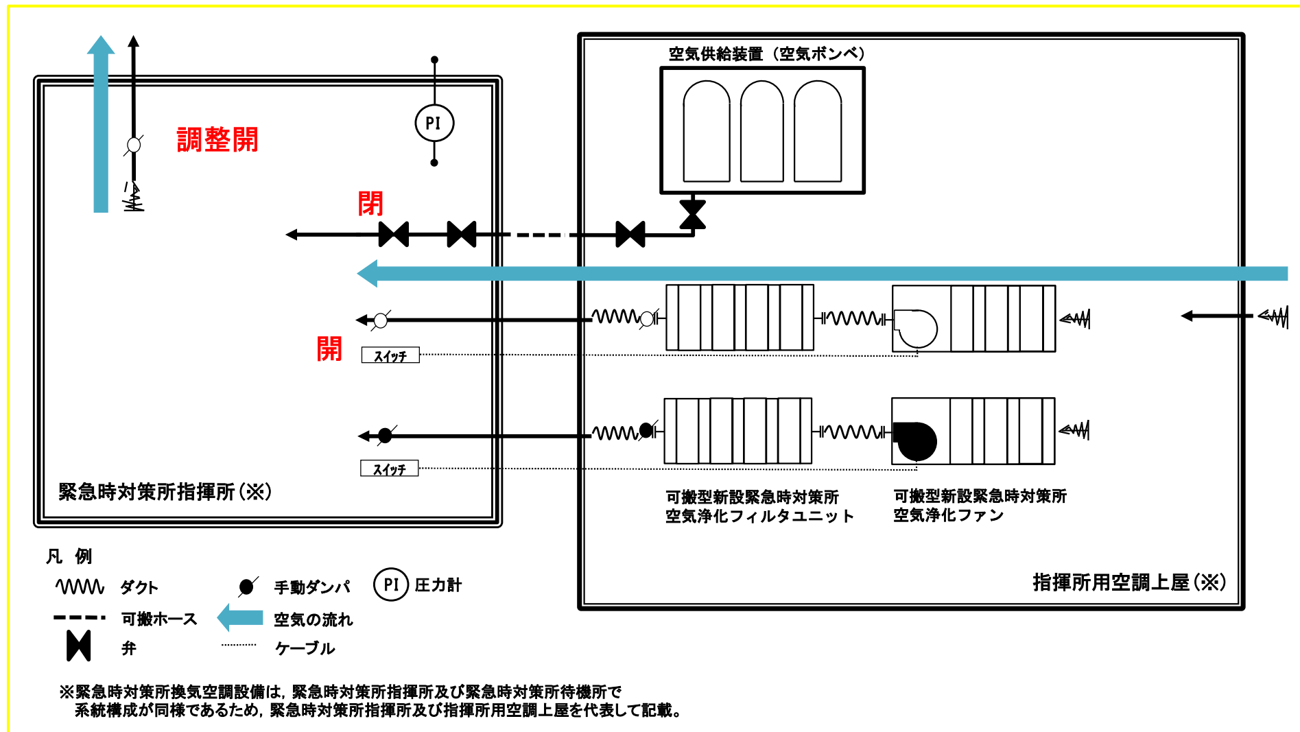
図11 緊急時対策所 換気設備 系統概略 (緊急時対策所立ち上げ時 (プルーム放出前まで))
