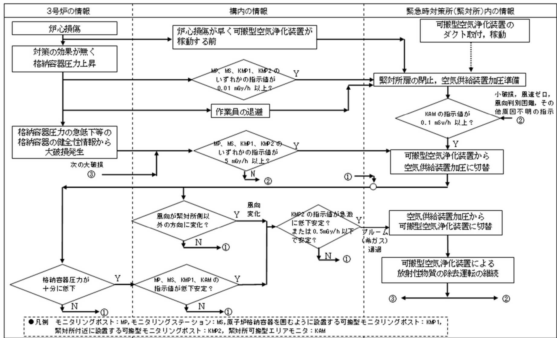
図14 緊急時対策所換気空調設備の運用基本フロー
