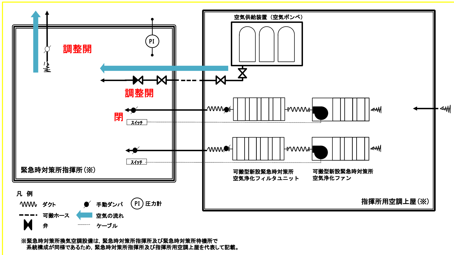
図12 緊急時対策所 換気設備 系統概略 (緊急時対策所立ち上げ時 (プルーム通過中))
