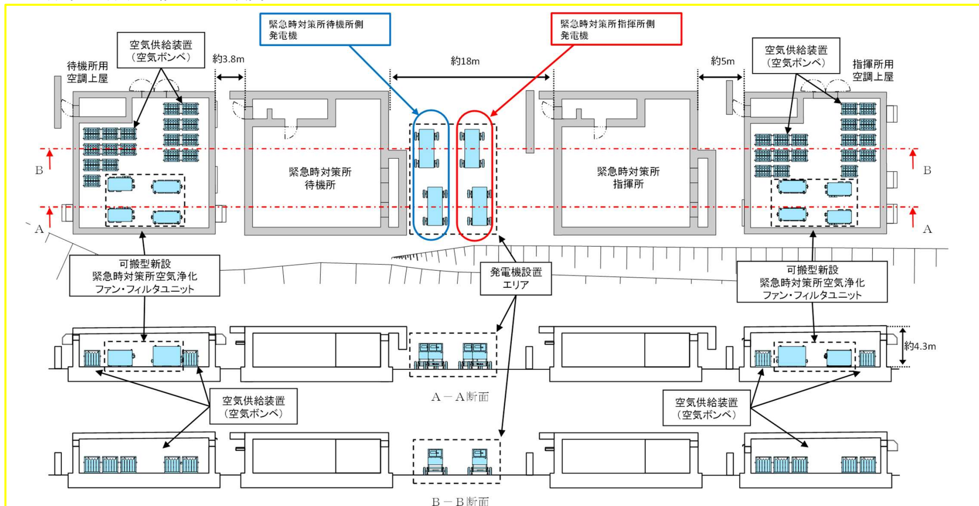
図2 緊急時対策所 周辺図
