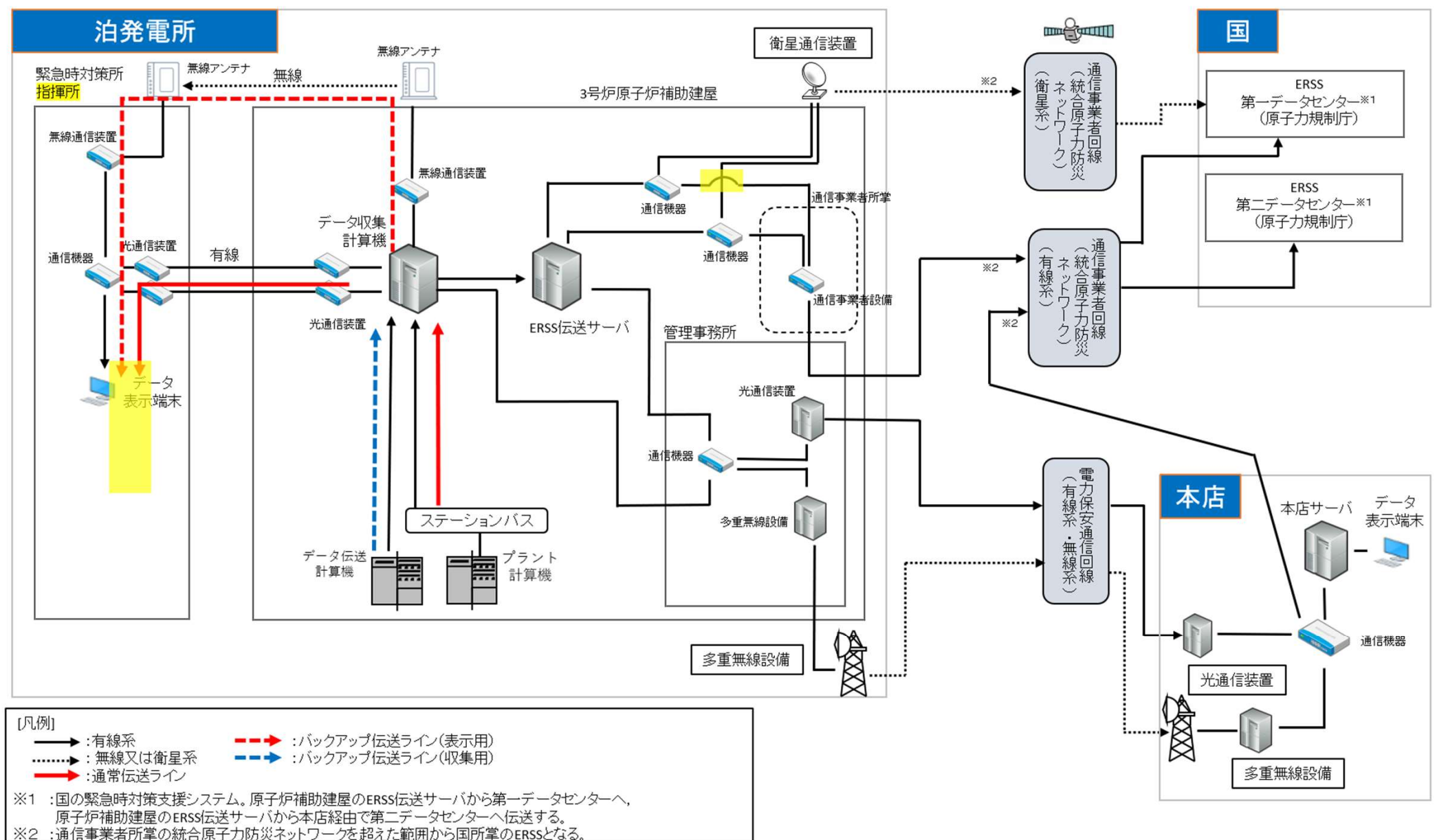
図5 緊急時対策所情報収集設備の概要
