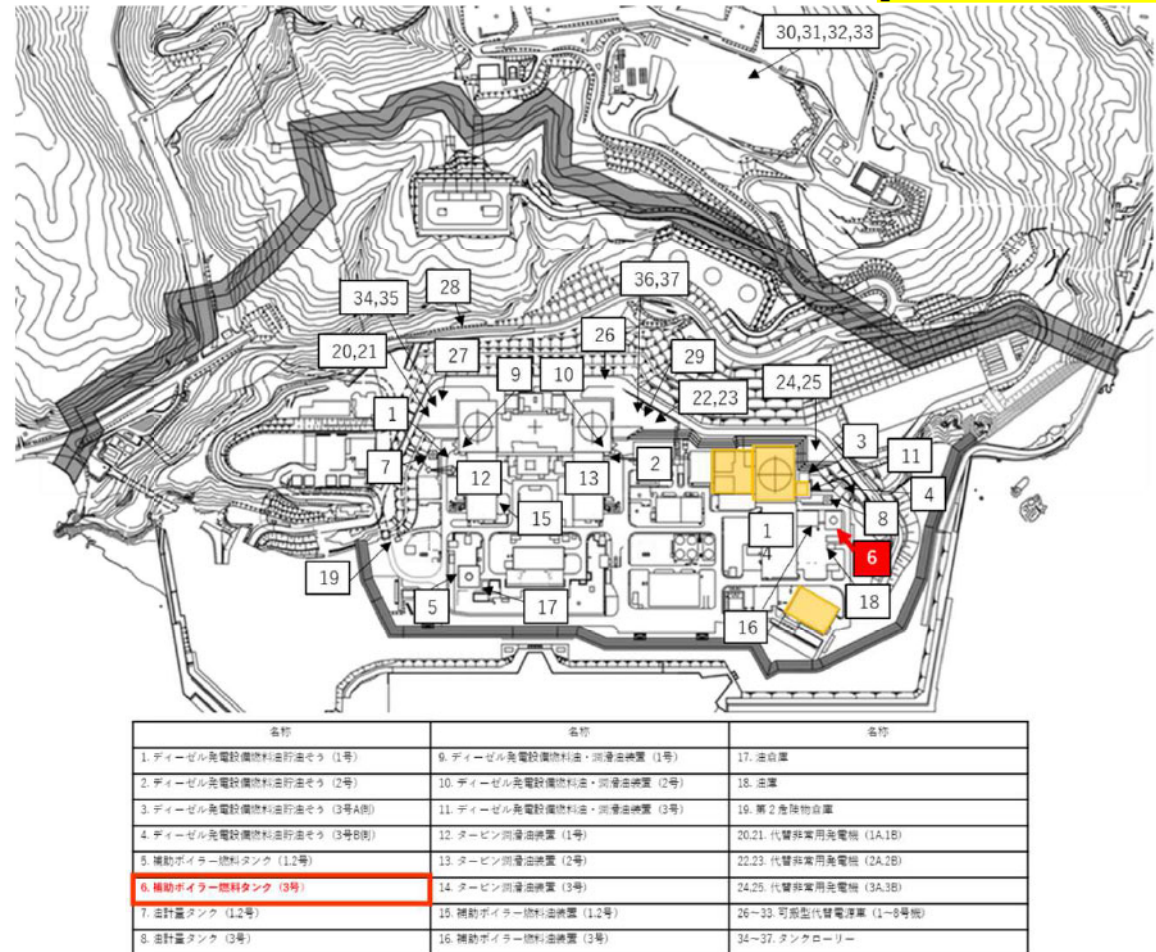
図6-2 敷地内における危険物施設の位置 (発電所全体)
