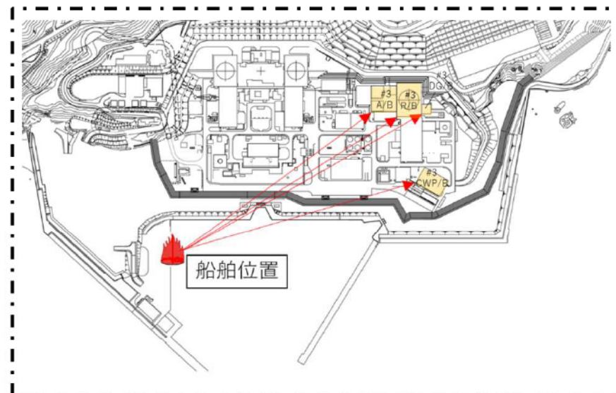
第2.2.4-1図 船舶火災想定位置と発電用原子炉施設との位置関係 [6-外火-別1-20]
