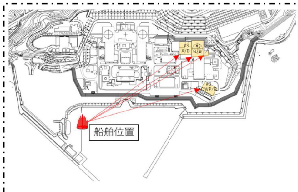
第2.2.4-1図 船舶火災想定位置と発電用原子炉施設との位置関係
