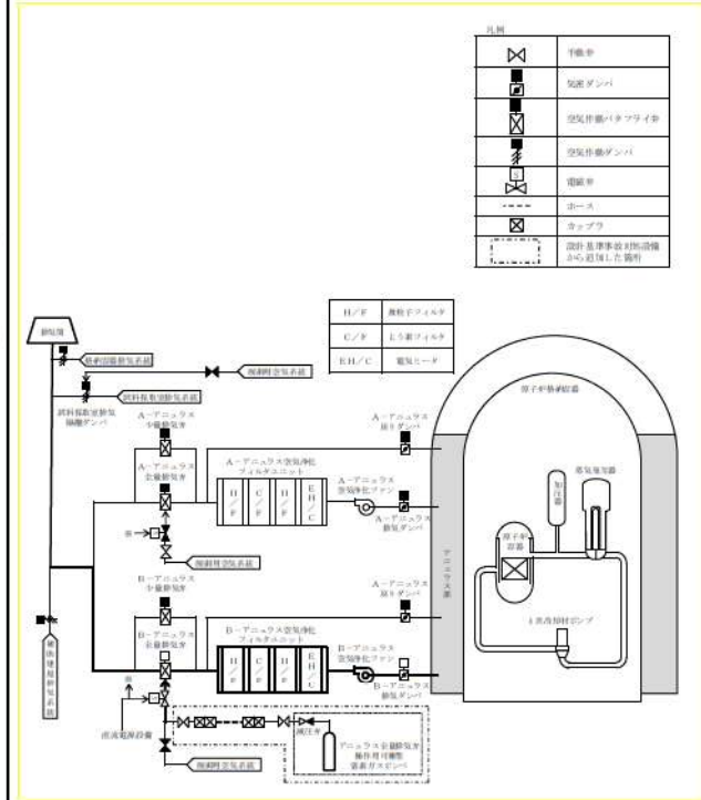
第1.16.14図 アニュラス空気浄化設備の運転
