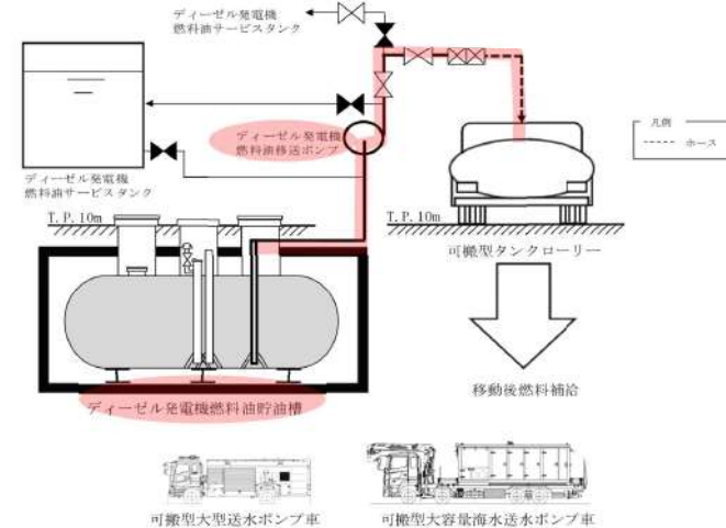
第10.2.10図 電源設備 概略系統図(11)
