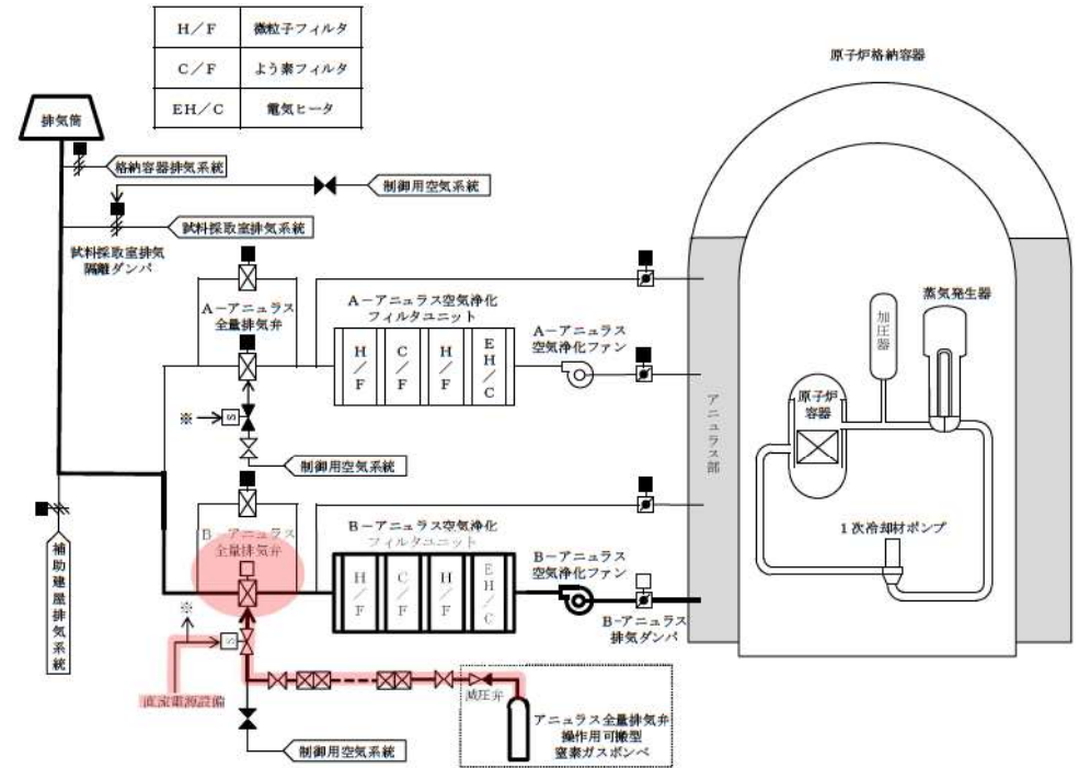
泊3号炉 水素爆発による原子炉建屋等の破損を防止するための設備 系統概要図
