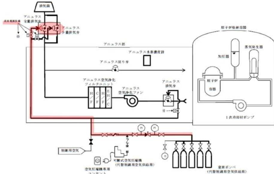
大飯3/4号炉 水素爆発による原子炉建屋等の破損を防止するための設備 系統概要図
