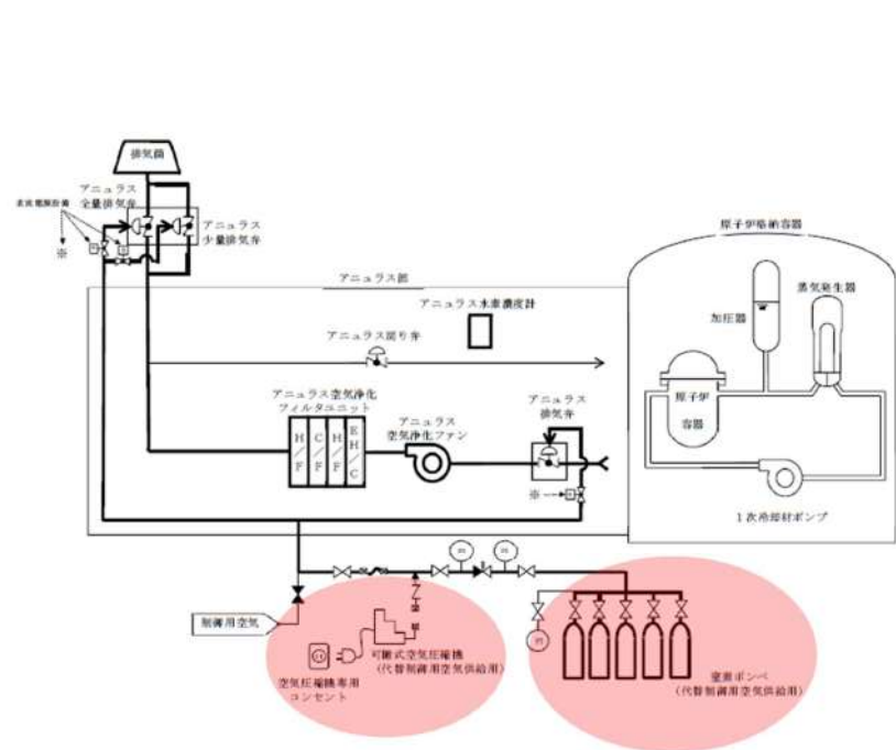
大飯3/4号炉 水素爆発による原子炉建屋等の破損を防止するための設備 概略系統図
