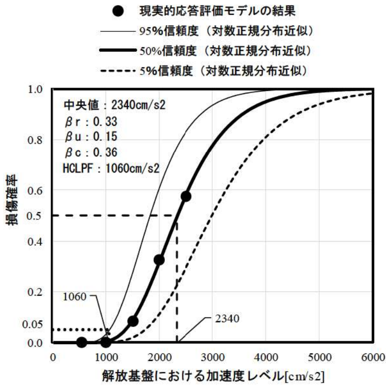
第 3.2.1. c-1-11 図 原子炉建屋のフラジリティ曲線 (NS 方向, 部材 6)
