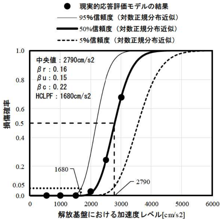
第 3.2.1. c-1-12 図 原子炉補助建屋のフラジリティ曲線 (EW 方向, 部材 9)
