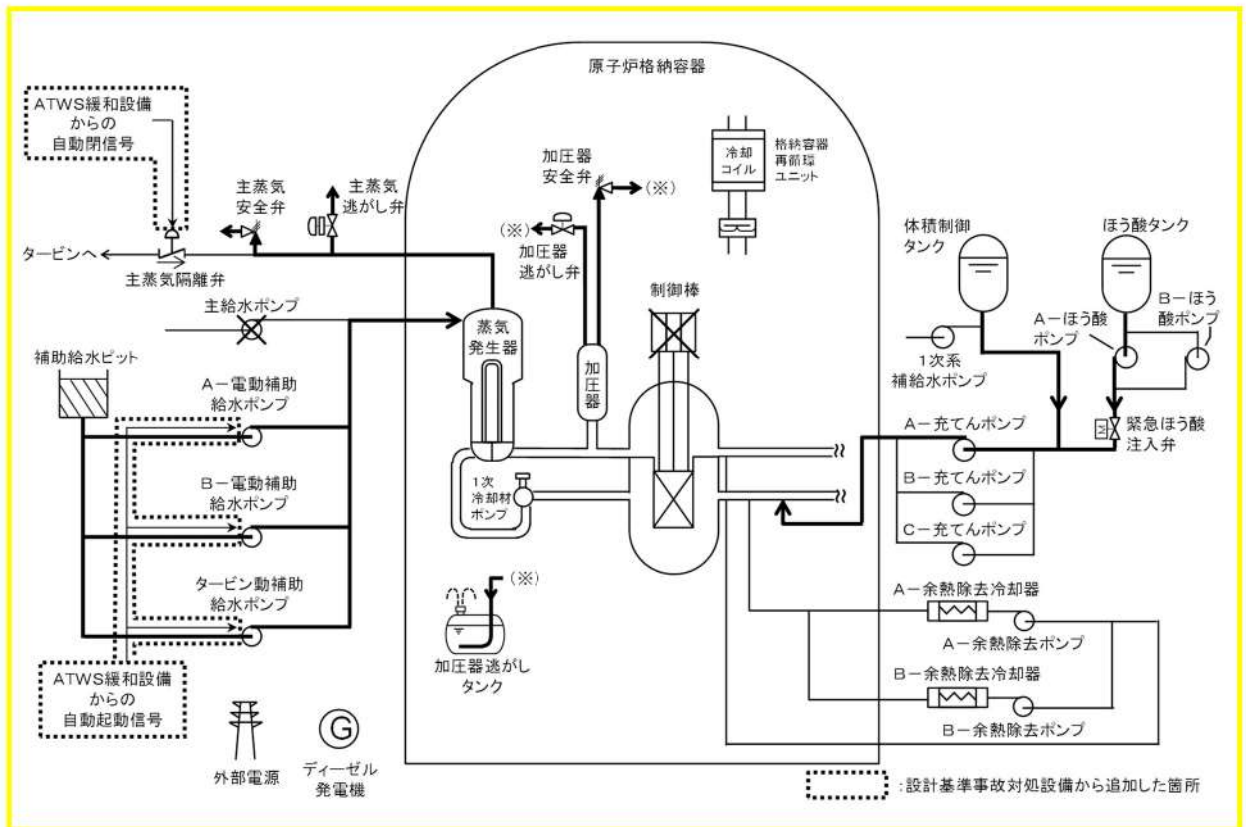
第 7.1.5.1 図 「原子炉停止機能喪失」の重大事故等対策の概略系統図（1 / 2） （ATWS 緩和設備及び緊急ほう酸濃縮）
