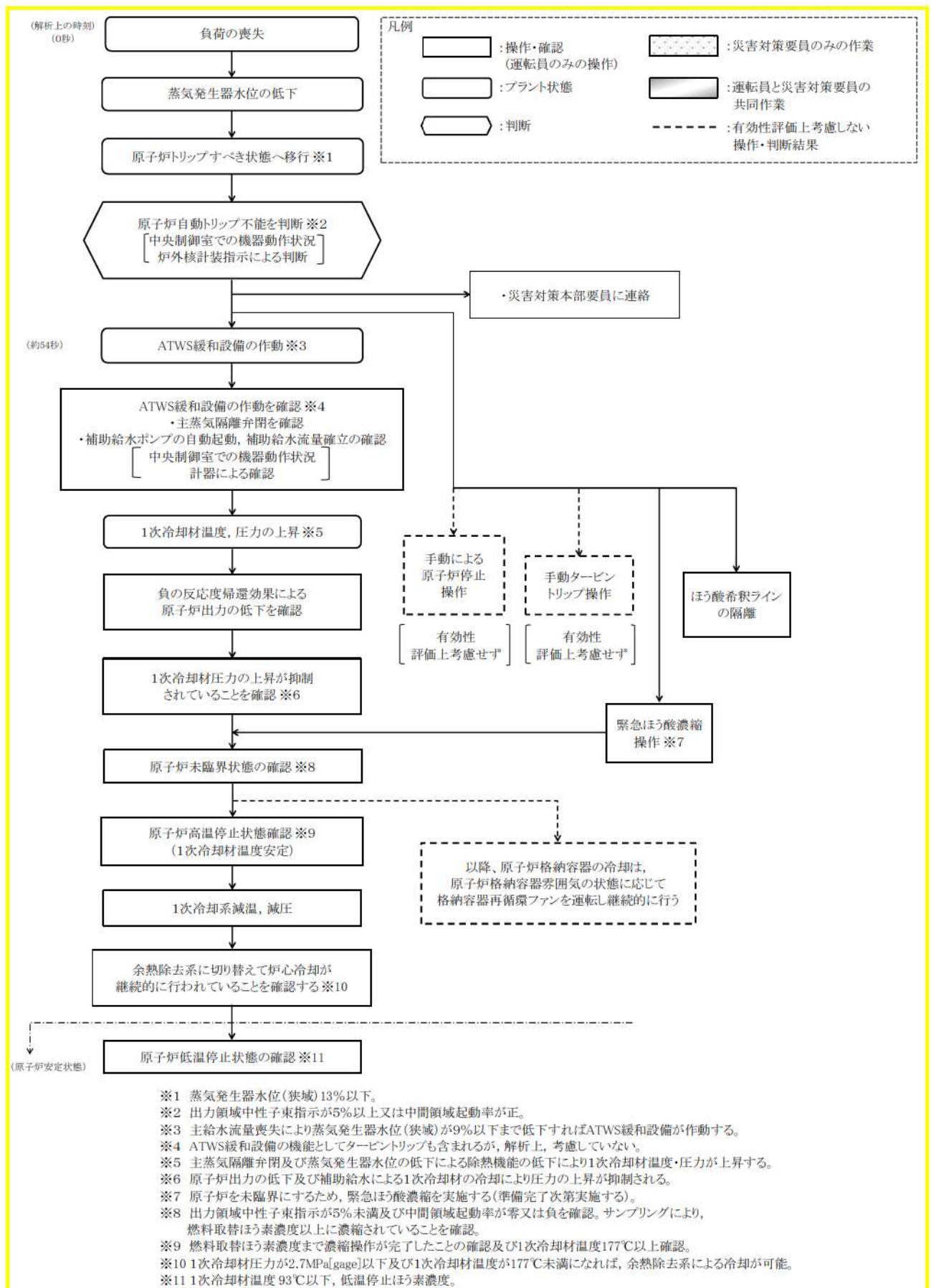
第 7.1.5.4 図 「原子炉停止機能喪失」の対応手順の概要 (「負荷の喪失時に原子炉トリップ機能が喪失する事故」の事象進展)
