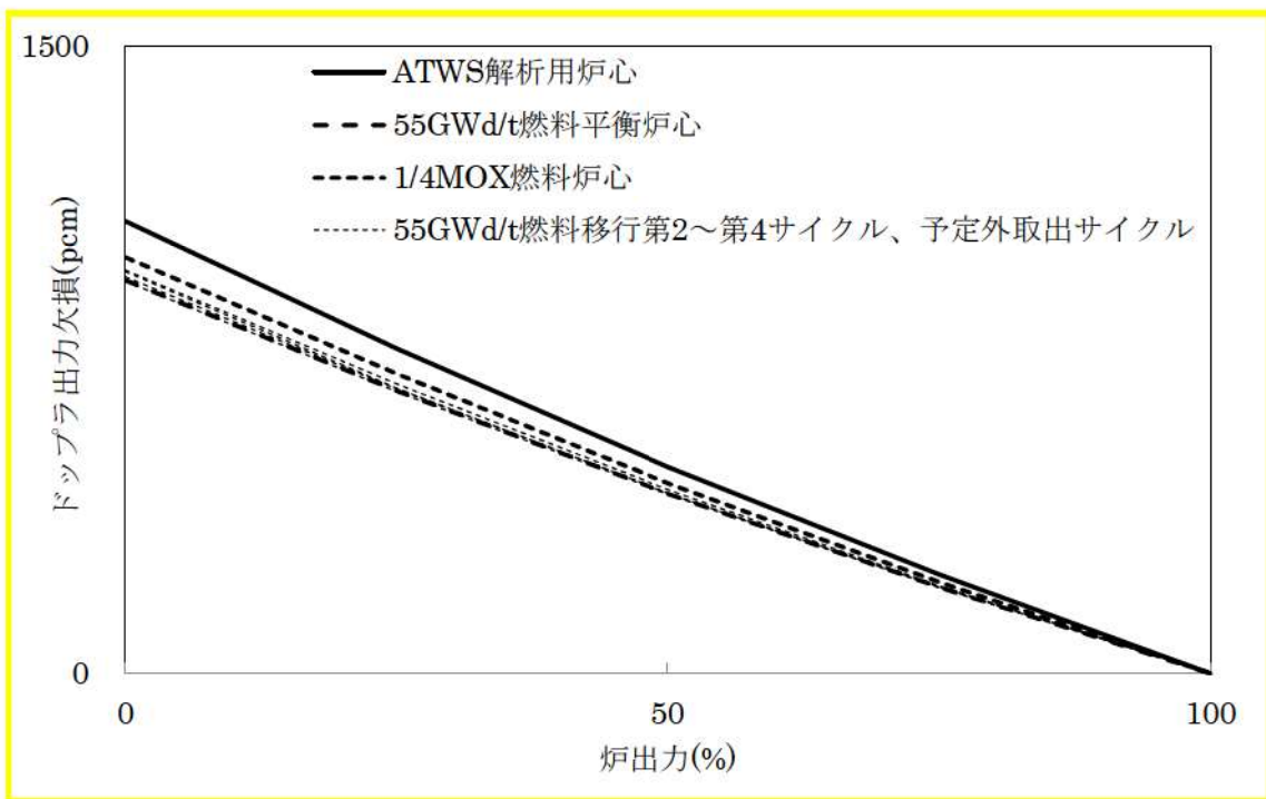
図4 ドップラ出力欠損
