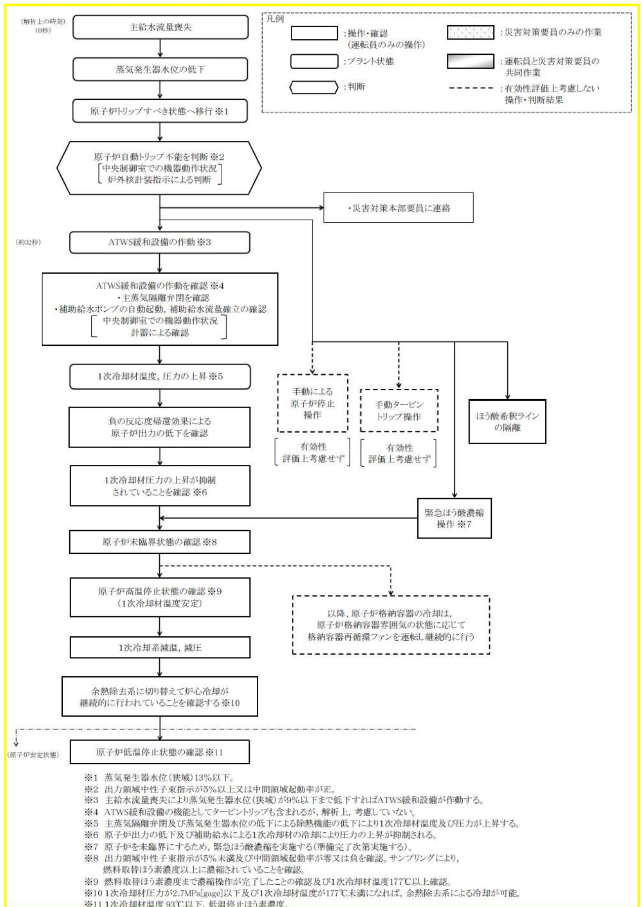
第 7.1.5.3 図 「原子炉停止機能喪失」の対応手順の概要 (「主給水流量喪失時に原子炉トリップ機能が喪失する事故」の事象進展)
