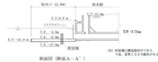
第 4.1-5 図 泊3号炉取水口付近詳細図
