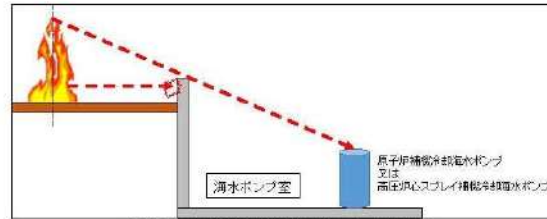
第6図 火災発生位置と海水ポンプの位置関係
