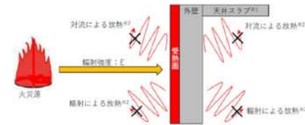
図4 一次元非定常熱伝導方程式による温度算出概念図
