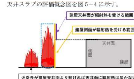
図5-4 建屋天井面の評価概念図
