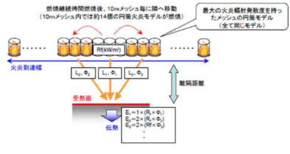
図 建屋の熱影響評価
