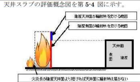
第5-4図 天井スラブの評価概念図
