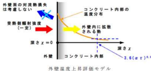
外壁温度上昇評価モデル
