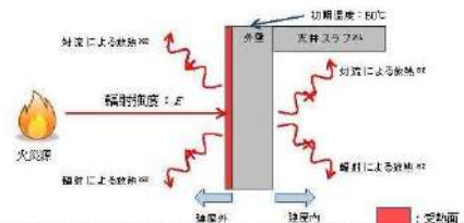
第9図 一次元非定常熱伝導方程式による温度算出概念図
