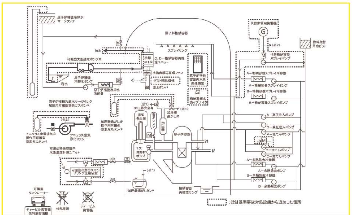
第 7.2.1.2.1 図 「雰囲気圧力・温度による静的負荷（格納容器過温破損）」 の重大事故等対策の概略系統図（2 / 2）（格納容器内自然対流冷却）
