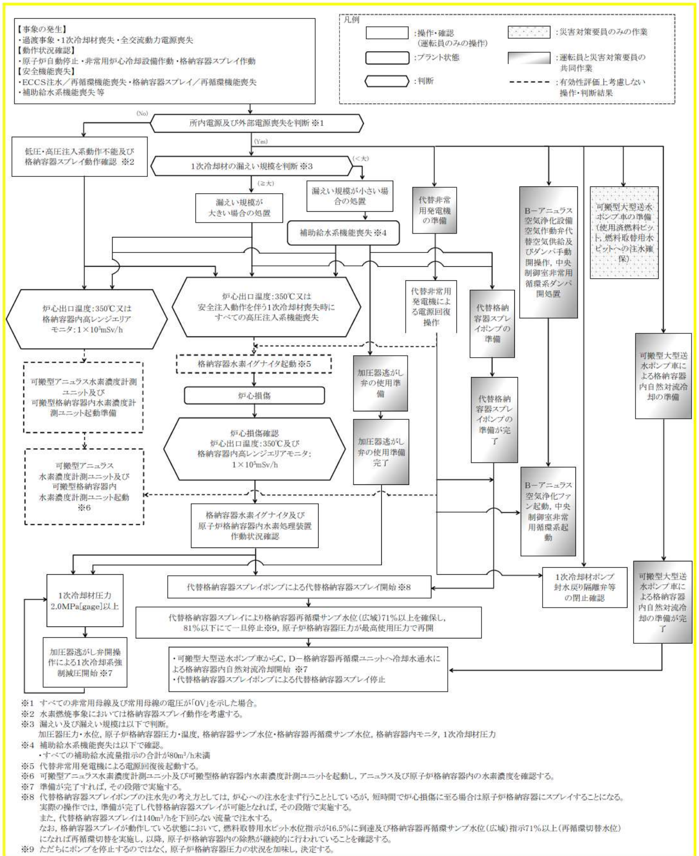
第 7. 2. 1. 2. 2 図 格納容器破損モード「雰囲気圧力・温度による静的負荷 (格納容器過温破損)」の対応手順の概要
