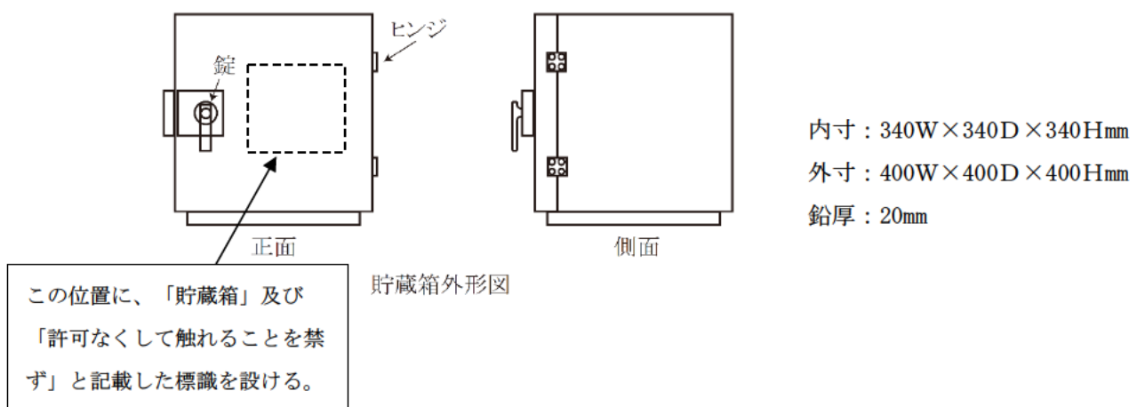
図4-3 アイソレーションルーム（I）内貯蔵施設 貯蔵箱の概略図
