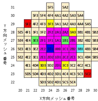
(C) 機械的エネルギーの解析(SIMMER-IV)の解析体系(炉心部)
