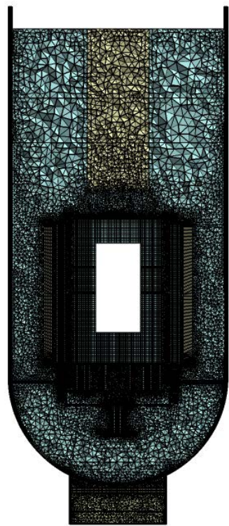
(3) 縦断面図
