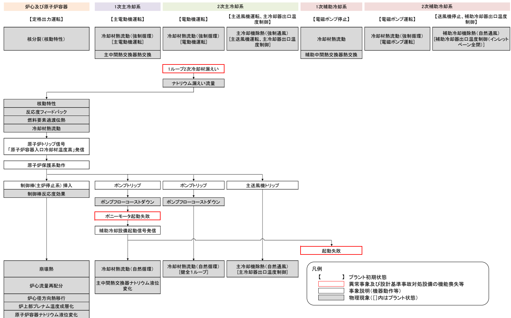
第6図 炉心損傷防止措置時 (PLOHS(ii)) の事象進展チャート
