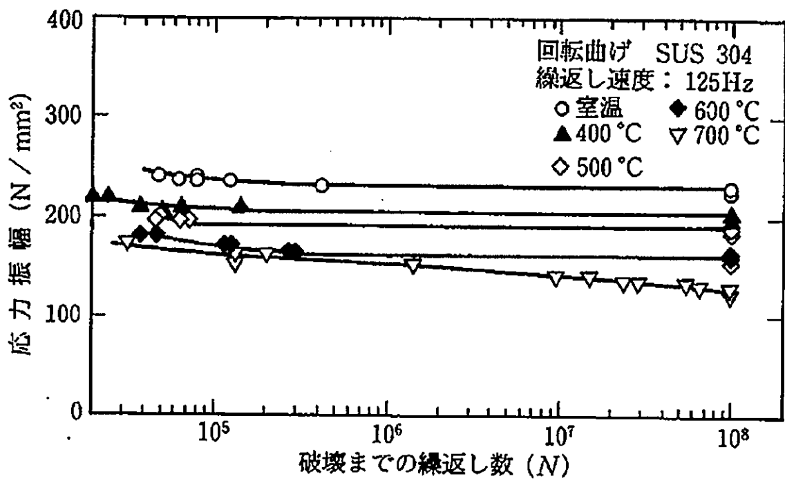
図(ロ)A-16 ステンレス鋼疲労曲線
