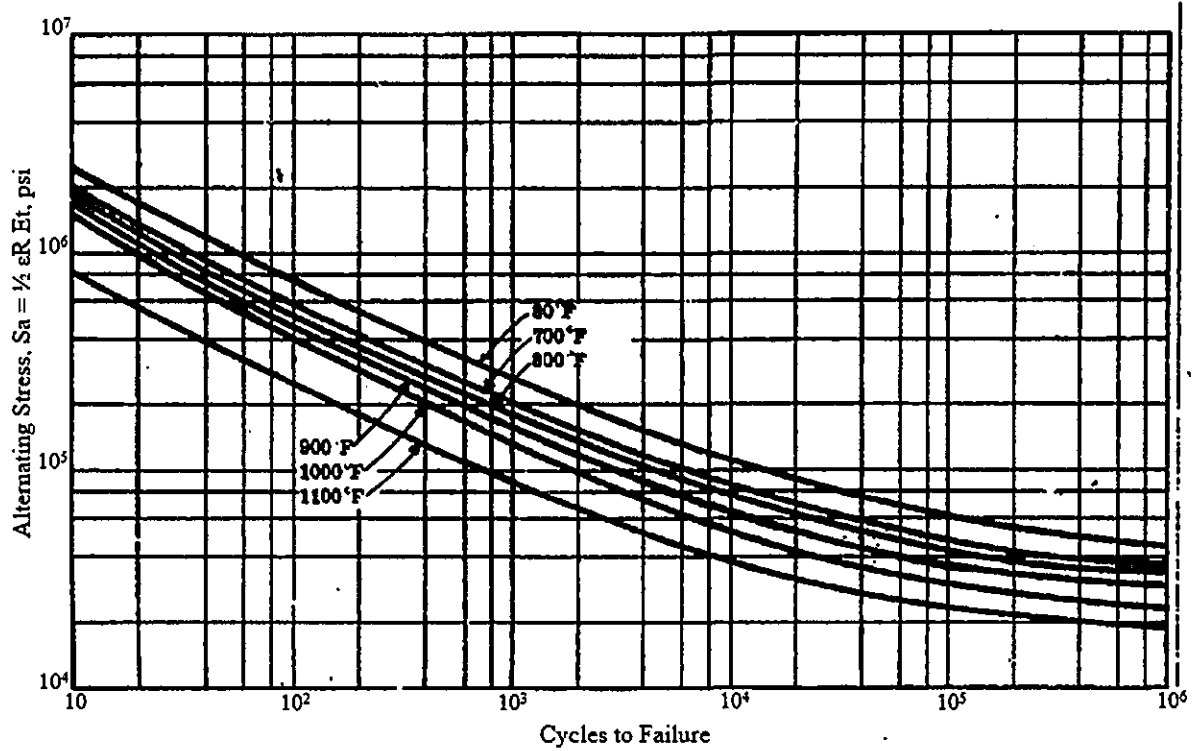
図(ロ)A-21 クロムモリブデン鋼疲労曲線
