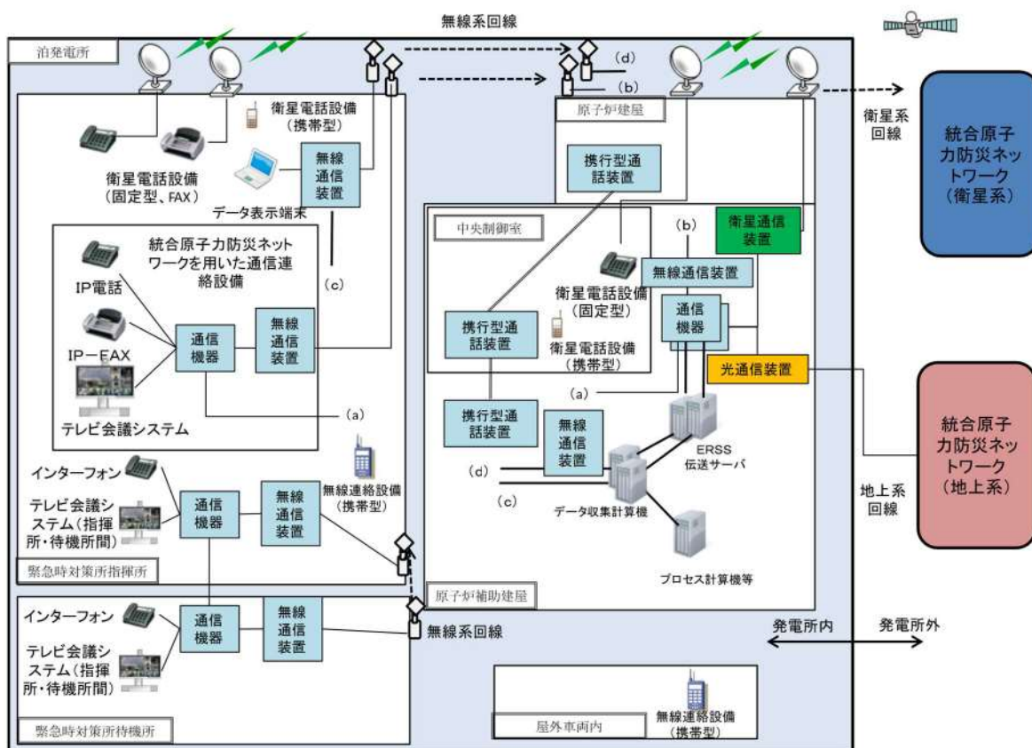
第 10.12-1 図 通信連絡設備系統概略図
