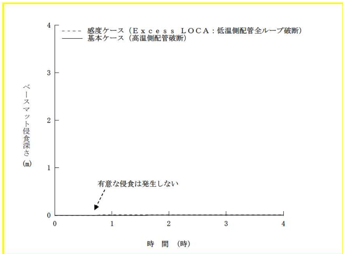
図10 ベースマット侵食深さ (壁面) の推移 (低温側配管全ループ破断時の影響確認)
