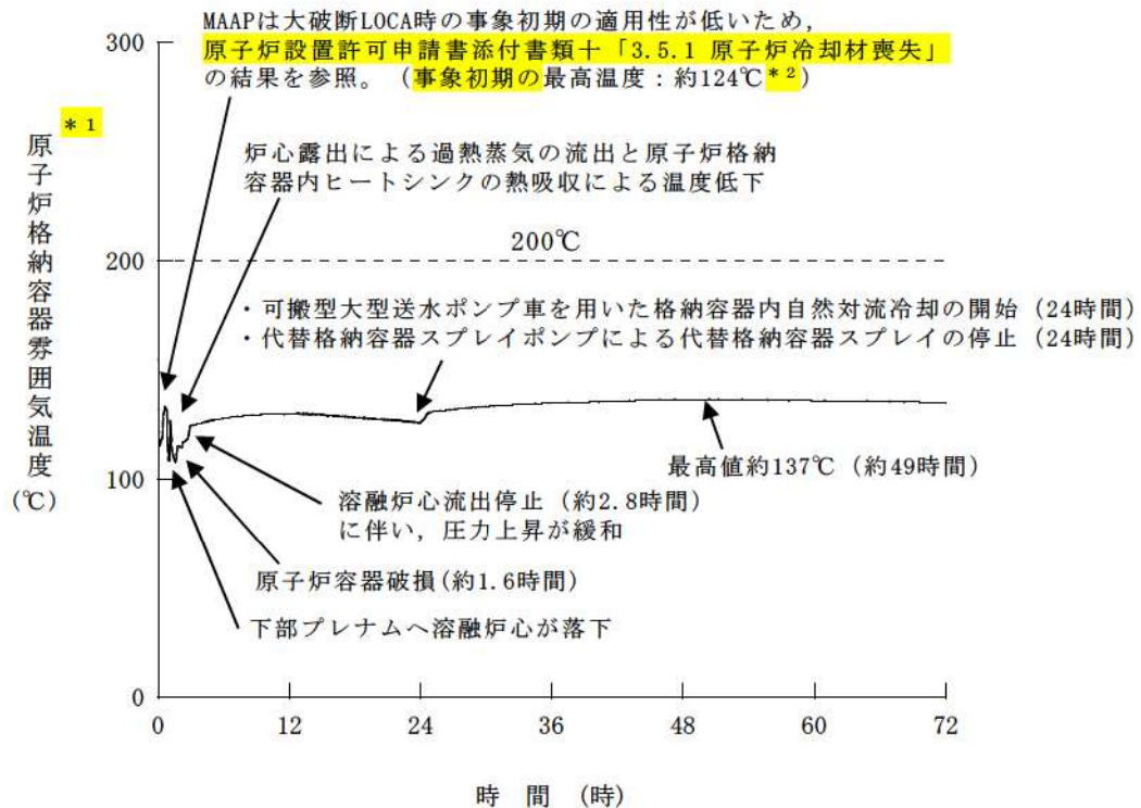
第 7.2.1.1.10 図 原子炉格納容器雰囲気温度の推移
