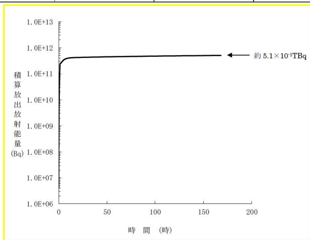
図1 Cs-137積算放出放射エネルギー(GROSS値)の推移（7日間(168時間)）
