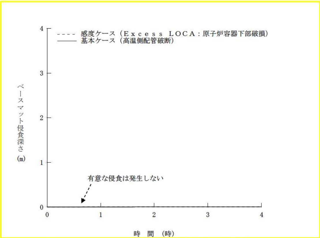
図 15 ベースマツト侵食深さ (壁面) の推移 (原子炉容器下端における破損時の影響確認)
