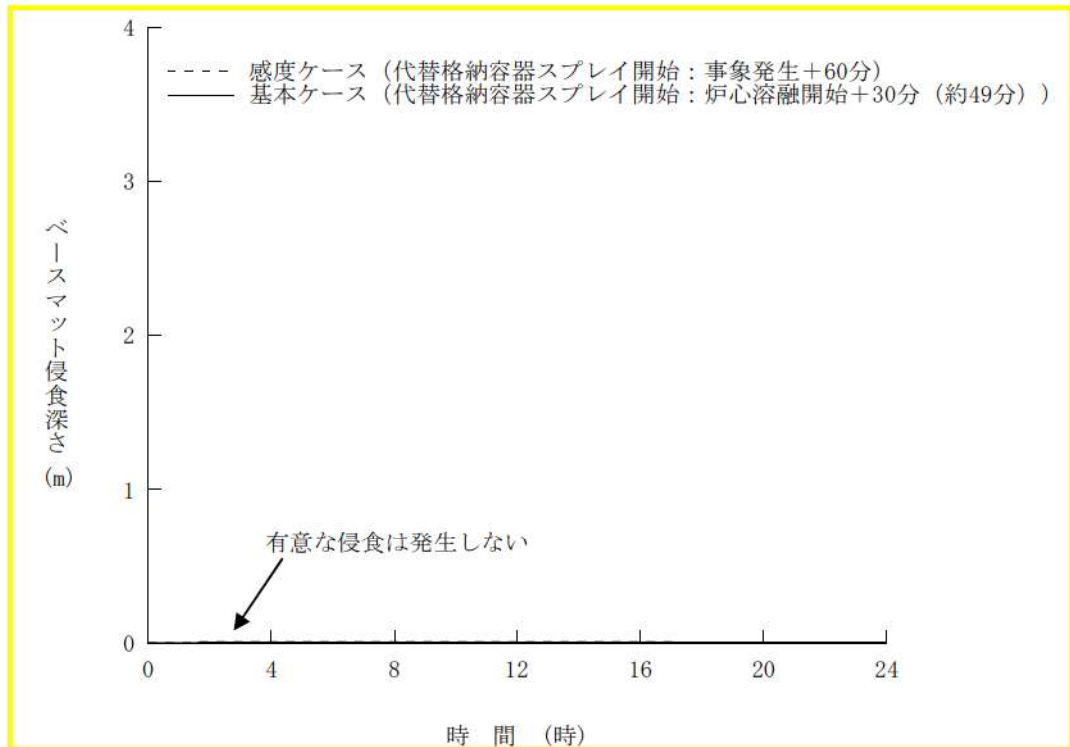
図5 ベースマット侵食深さ (床面) の推移 (代替格納容器スプレイ操作時間余裕確認)
