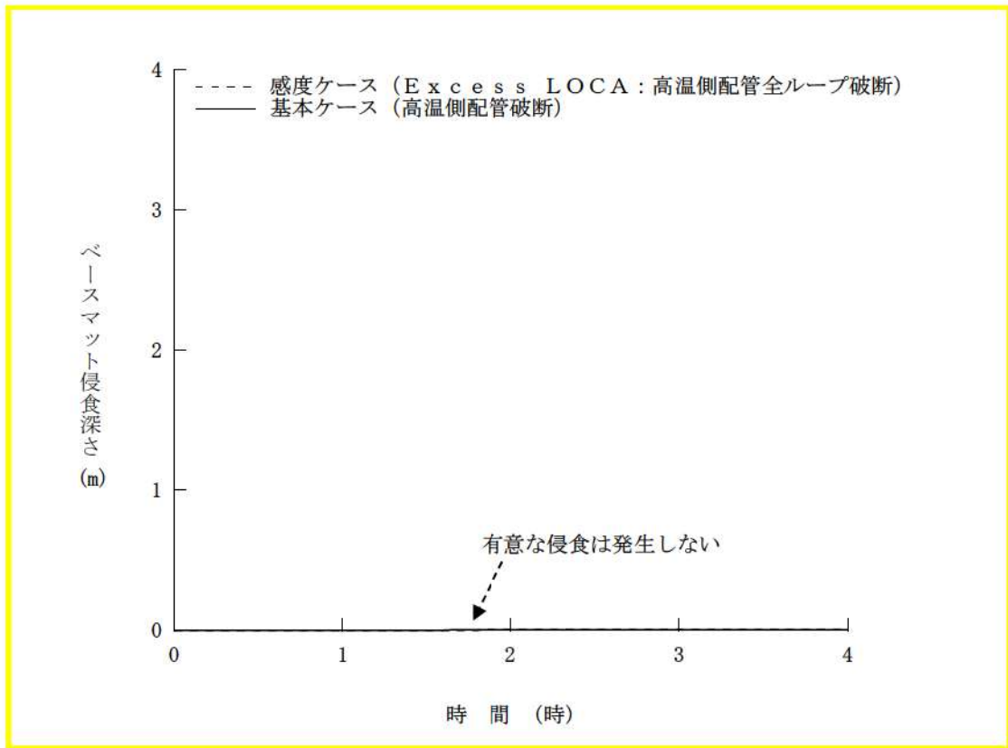
図5 ベースマット侵食深さ（壁面）の推移 （高温側配管全ループ破断時の影響確認）
