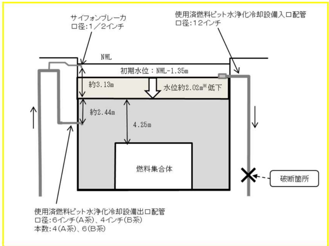
使用済燃料ピット水位概要図
