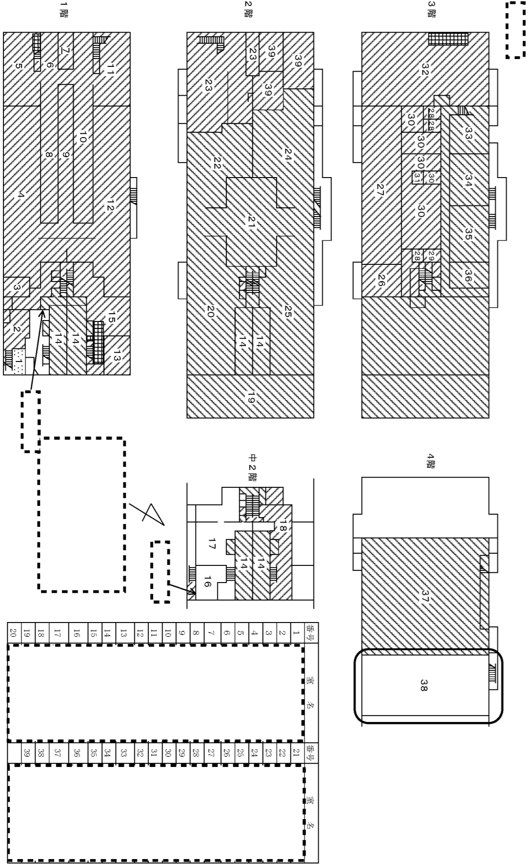
別図2-1(3) 管理区域及びV 1 保全区域図
