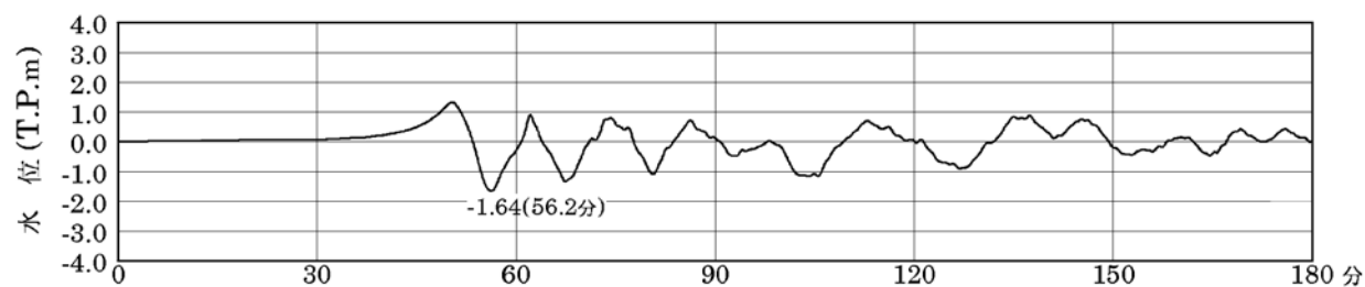
第1.2-9図(4) 基準津波の取水口位置での時刻歴波形 (初期潮位:T.P.±0.00m)
