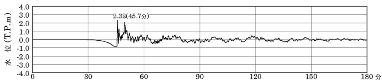
第1.2-9図(3) 基準津波の取水ピット前面位置での時刻歴波形 (初期潮位:T.P.±0.00m)
