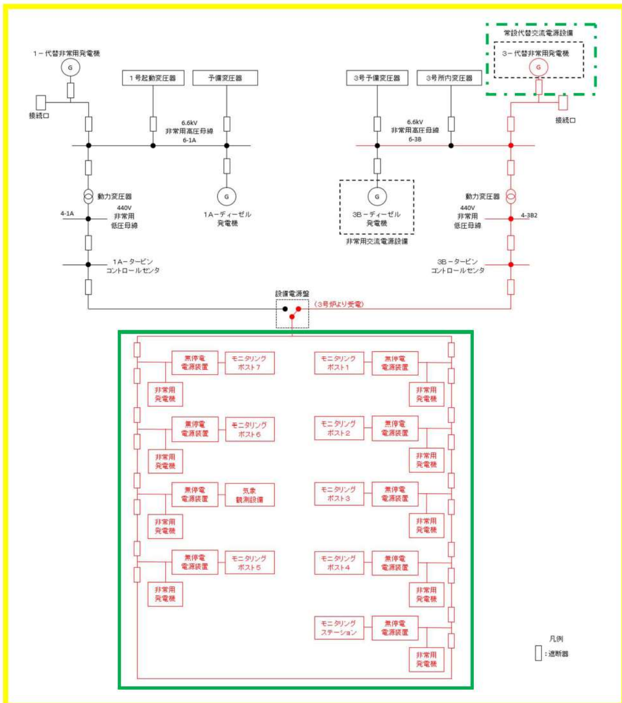
第 1.1.2-1 図 モニタリングポスト及びモニタリングステーションの電源構成概略図等 (1/2)
