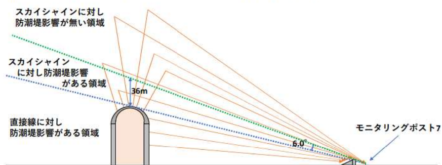
第6図 直接・スカイシャイン線の経路
