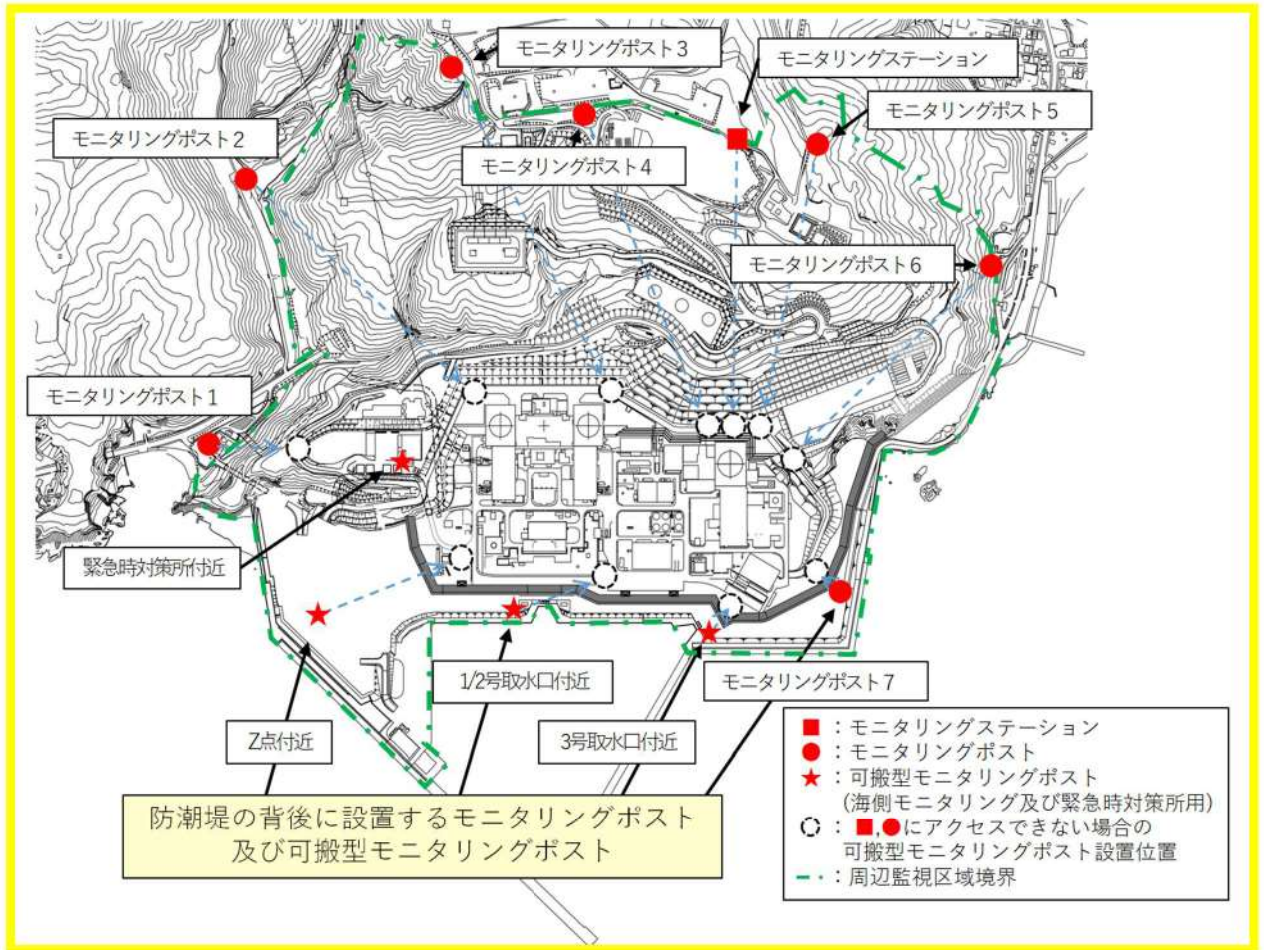
第1図 防潮堤の背後に設置するモニタリングポストおよび可搬型モニタリングポスト配置
