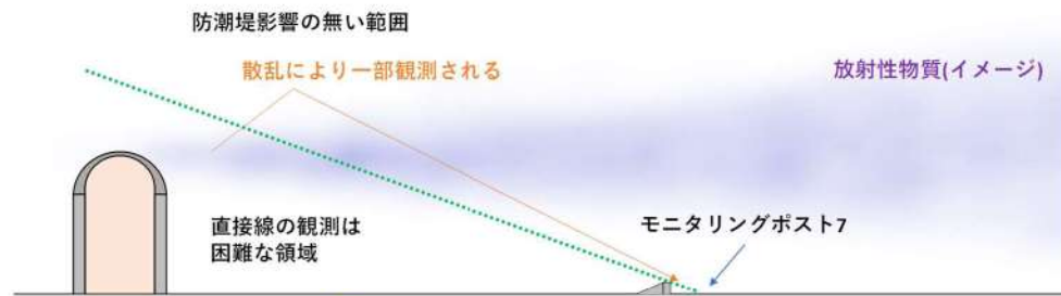
第5図 クラウドシャイン線の観測
