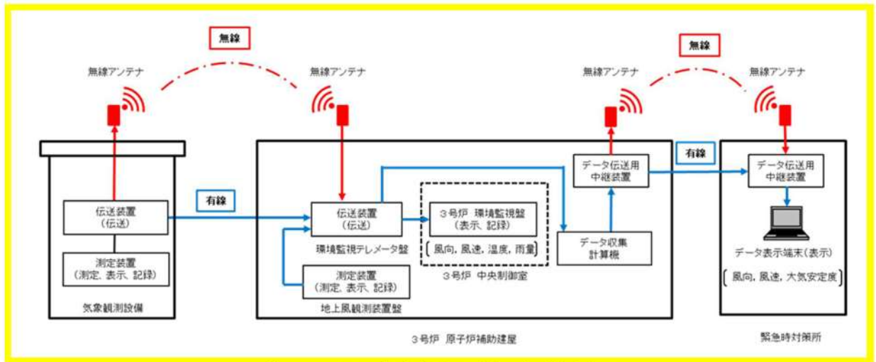
第 2.1-2 図 気象観測設備の伝送概略図
