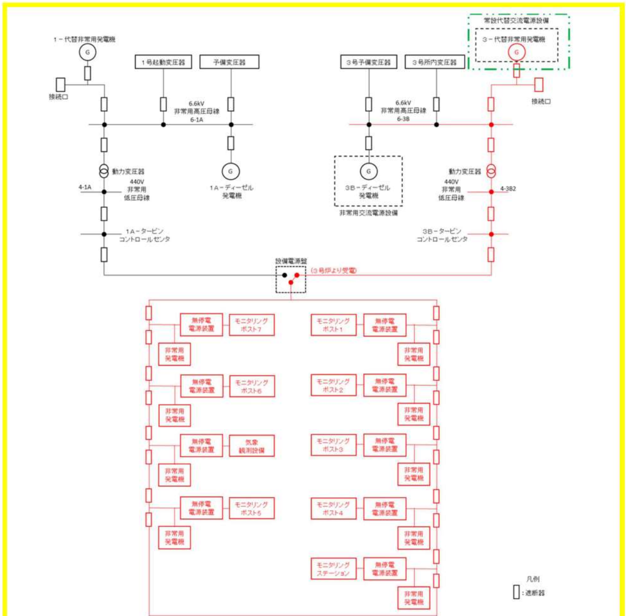
第1図 モニタリングポスト及びモニタリングステーションの電源構成概略図
