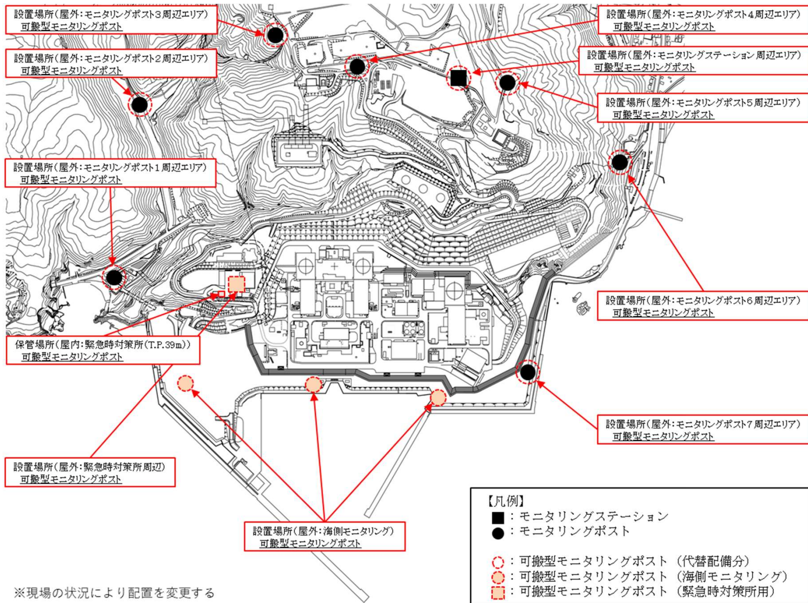
図4 可搬型モニタリングポスト 設置場所及び保管場所図
