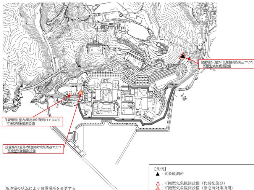
図5 可搬型気象観測設備 設置場所及び保管場所図
