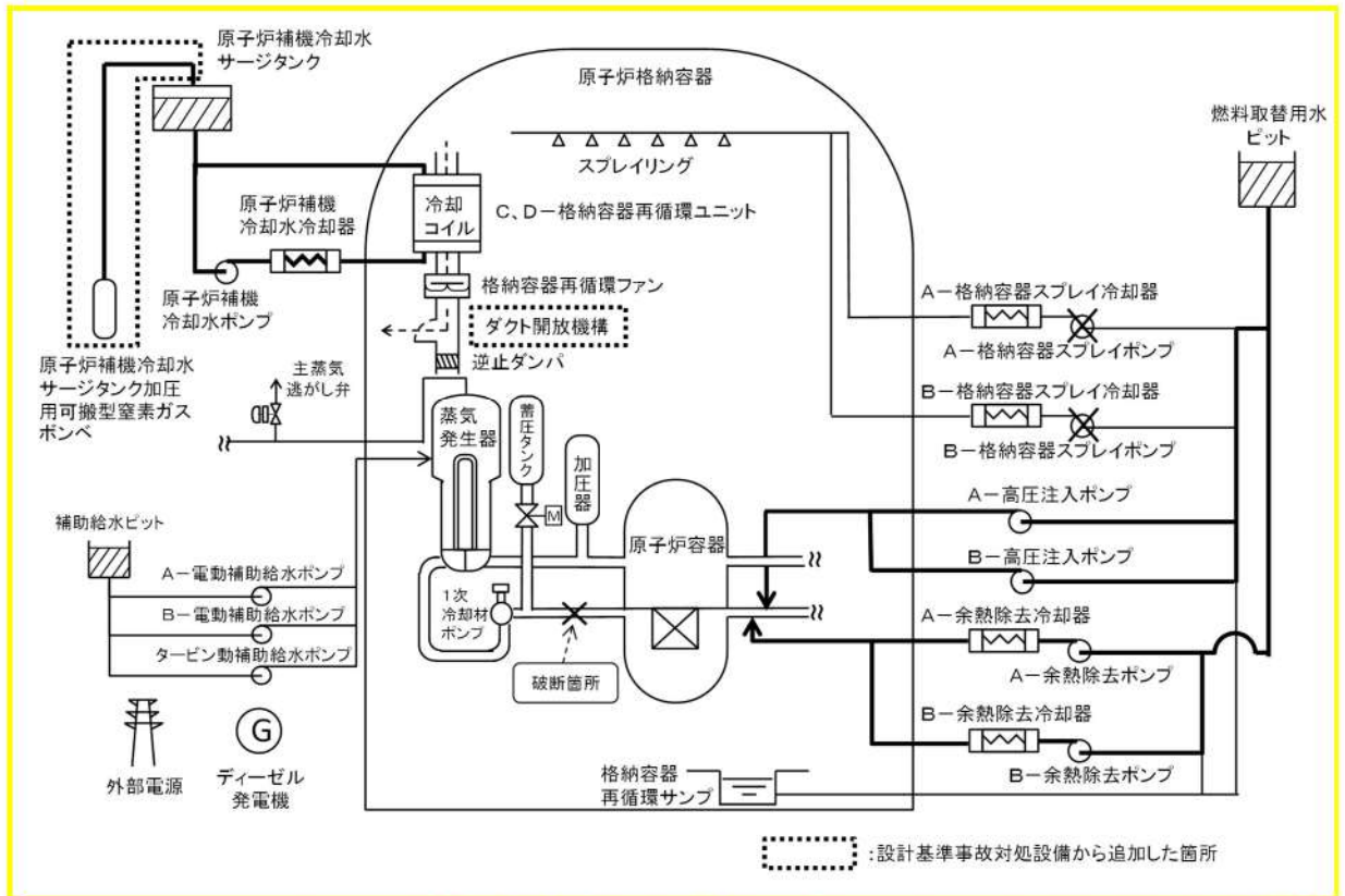
第 7.1.4.1 図 「原子炉格納容器の除熱機能喪失」の重大事故等対策の概略系統図 (1/2) (高圧注入, 低圧注入及び格納容器内自然対流冷却)
