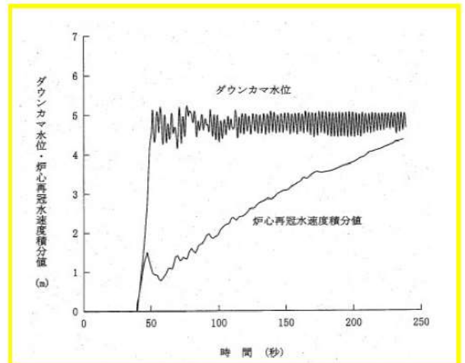
図2 ECCS性能評価解析 (DBA) の結果 (ダウンカマ水位、炉心再冠水速度積分値) (設置変更許可添付書類十と同じ)
