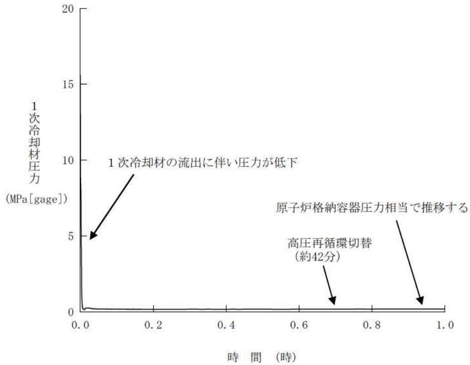
図1 1次冷却材圧力の推移 (本資料 第7.1.4.4図の拡大図)
