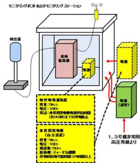
第 1.1.2 図 モニタリングポスト及びモニタリングステーションの電源構成概略図等 (2/2)
