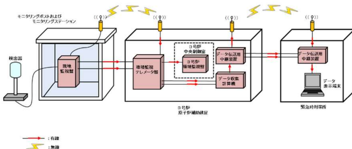
第 1.1.3 図 モニタリングポスト及びモニタリングステーション設備の伝送概略図
