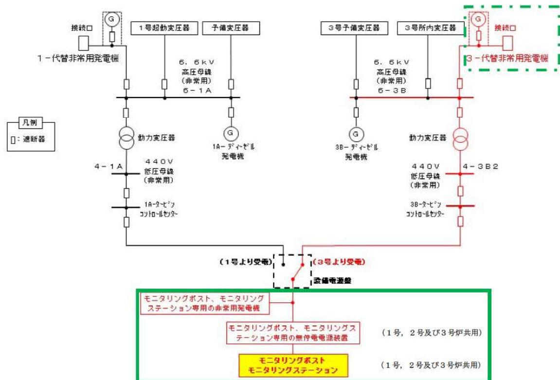
第 1.1.2 図 モニタリングポスト及びモニタリングステーションの電源構成概略図等 (1/2)
