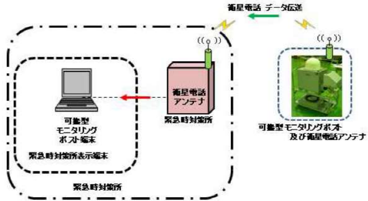
第 1.3.1-2 図 可搬型モニタリングポストの伝送概略図
