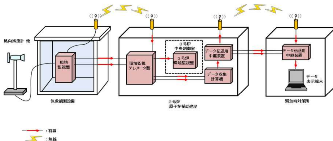
第 2.1-2 図 気象観測設備の伝送概略図
