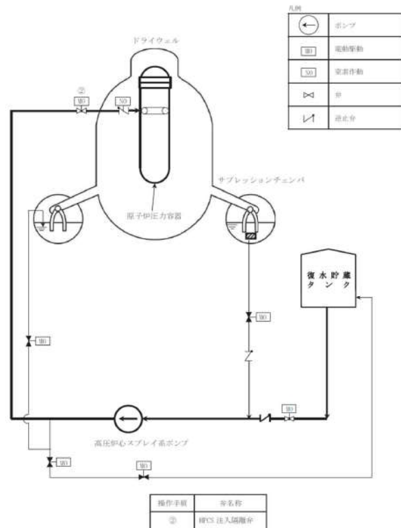
第1.2-18図 高圧炉心スプレイ系による原子炉圧力容器への注水 概要図(1/2) (高圧炉心スプレイ系による原子炉圧力容器への注水)
