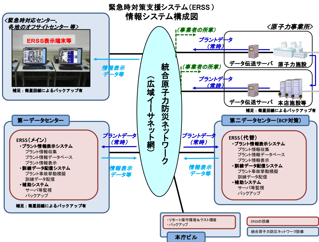
図1 現行ERS Sのシステム概要図
