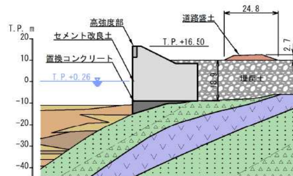
地質断面図 (6-6')
