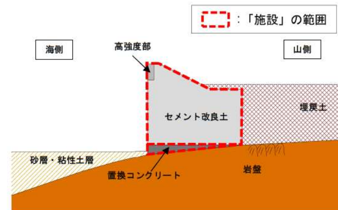
防潮堤断面図(既設護岸及び埋戻土がない状態)
