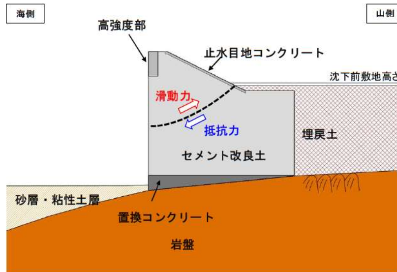
すべり線のイメージ図
