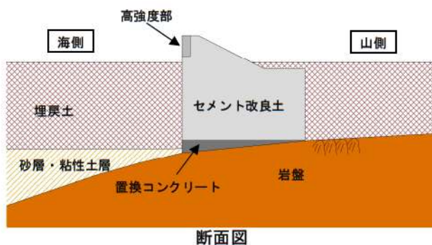
断面図 防潮堤（標準部）
