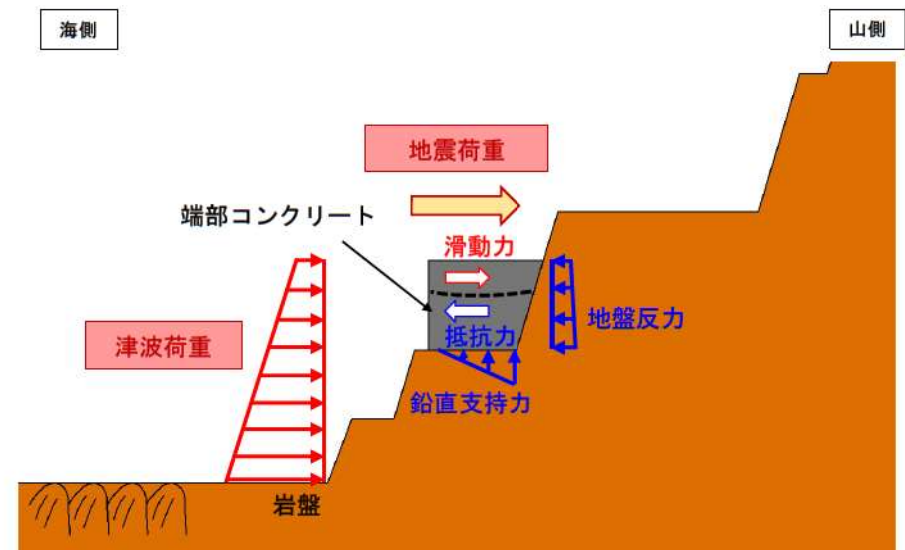
荷重図
