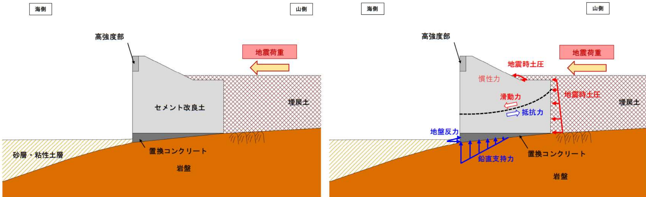
変形モード (防潮堤に生じる変位は小さい)
