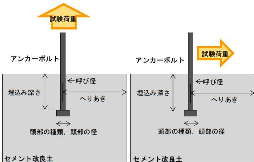
引張試験イメージ図
