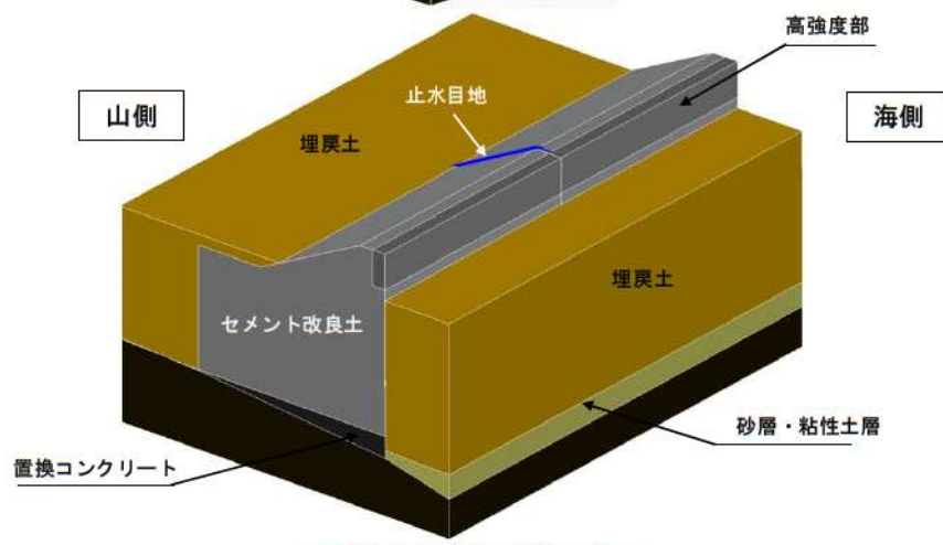
防潮堤(標準部)の構造概要
