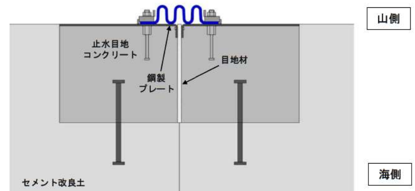
防潮堤(標準部) 屈曲部以外の施工目地 構造概要
