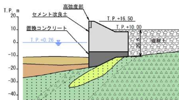
地質断面図 (2-2')
