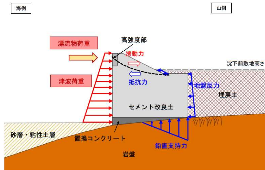
荷重図
