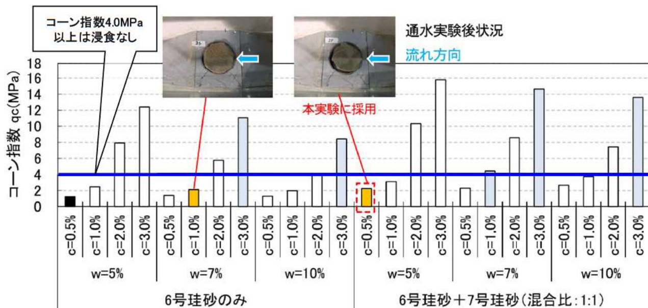
実験結果(一部追記)
