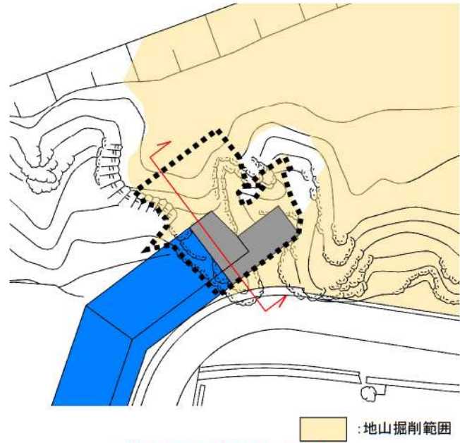
防潮堤掘削側端部(掘削前)
