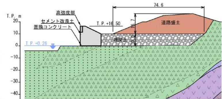
地質断面図 (7-7')
