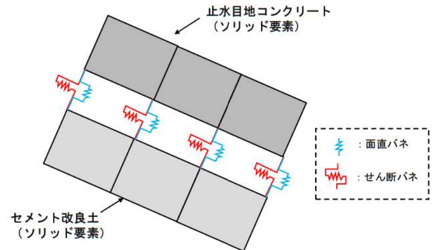
止水目地コンクリートとセメント改良土の境界部のモデル化イメージ図
