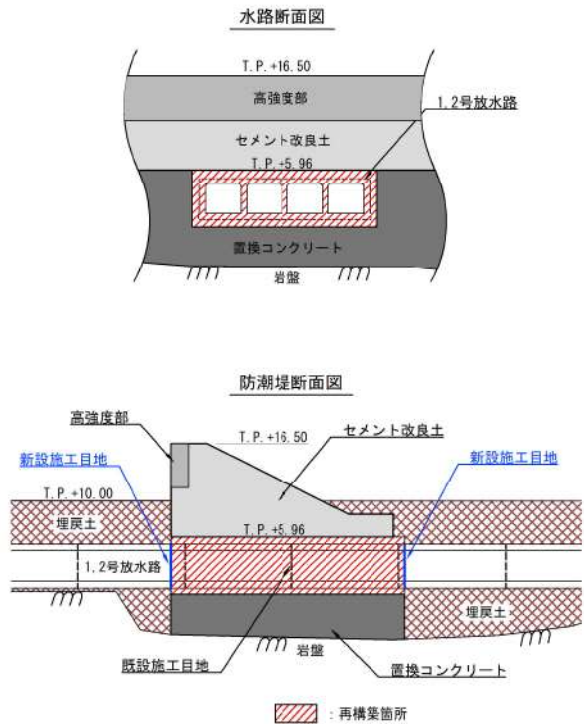
1,2号放水路横断面部
