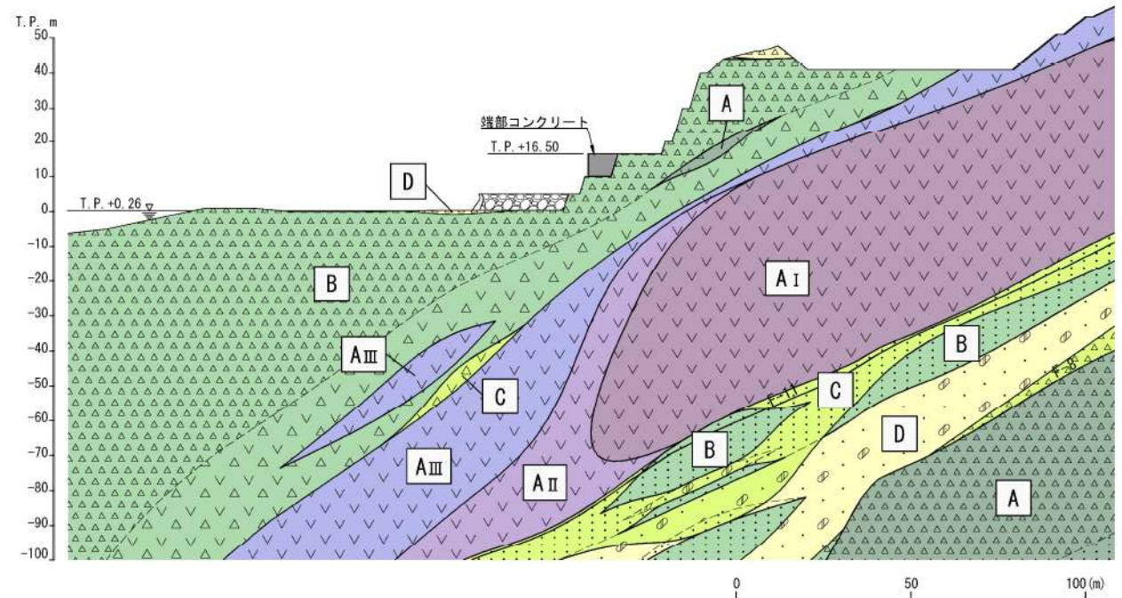
地質断面図 (8-8')
