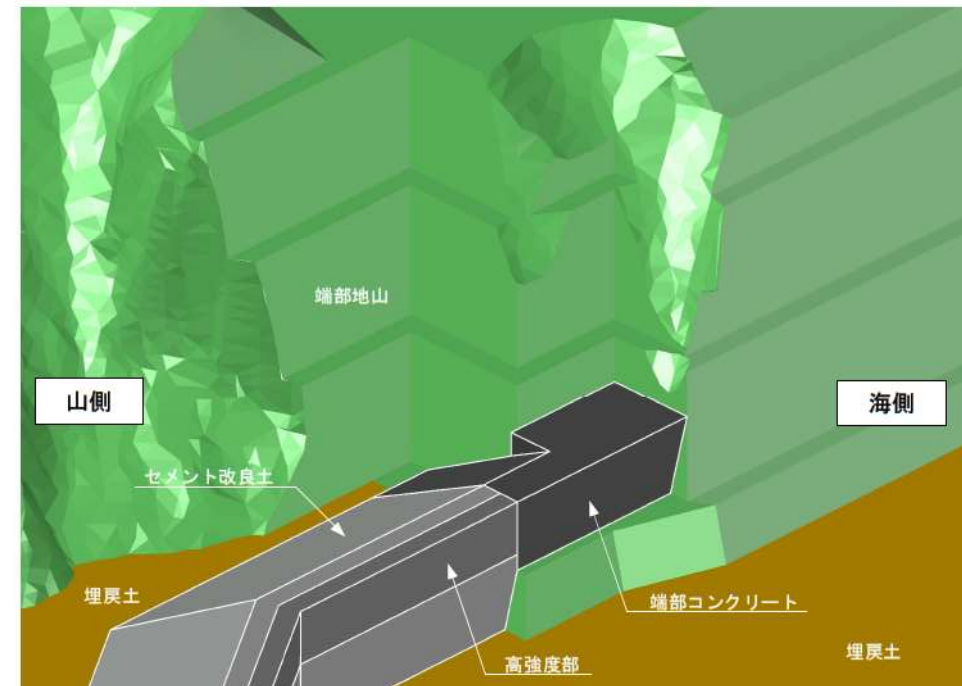
防潮堤(端部)の構造イメージ図
