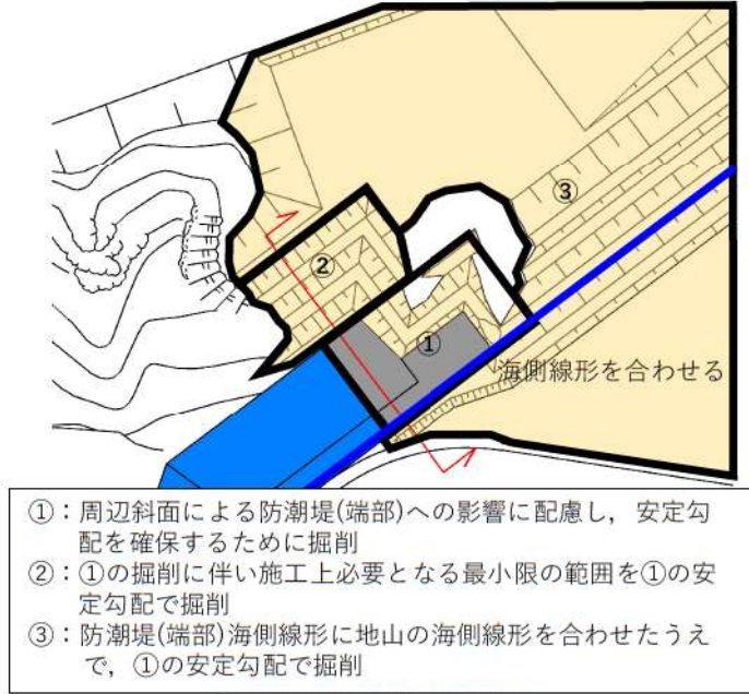
防潮堤掘削側端部(掘削後)
