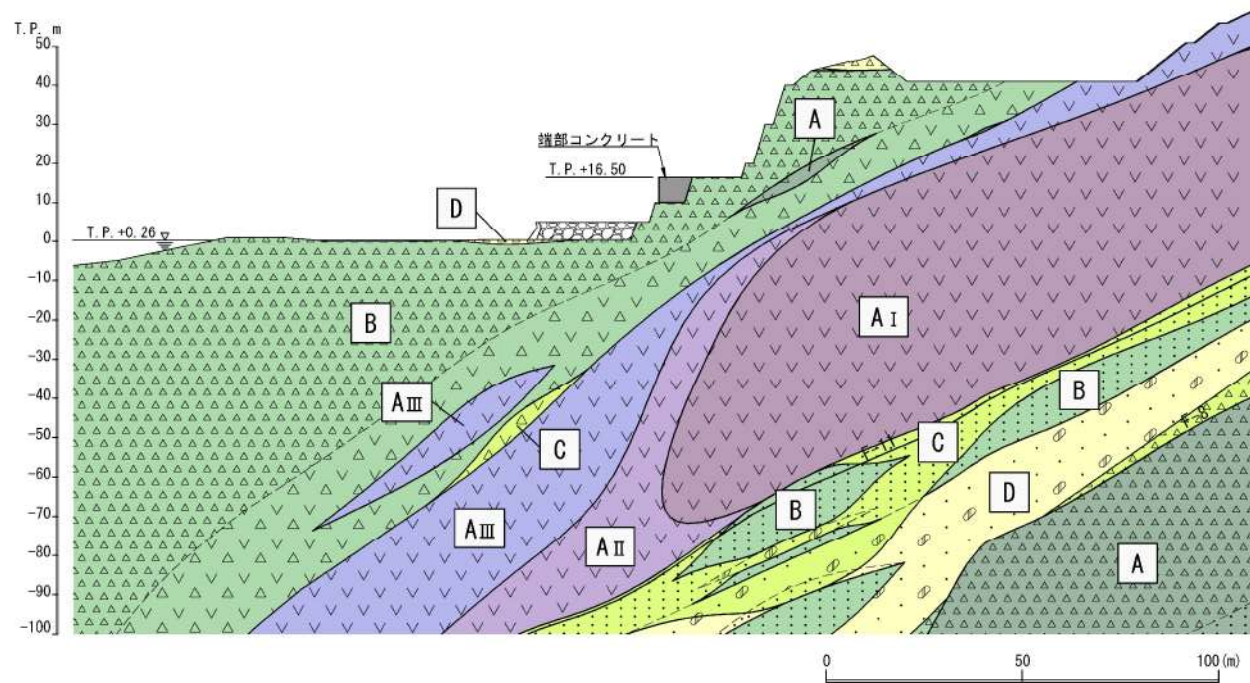
地質断面図(8-8')
