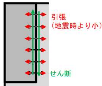
アンカーボルトの作用力
