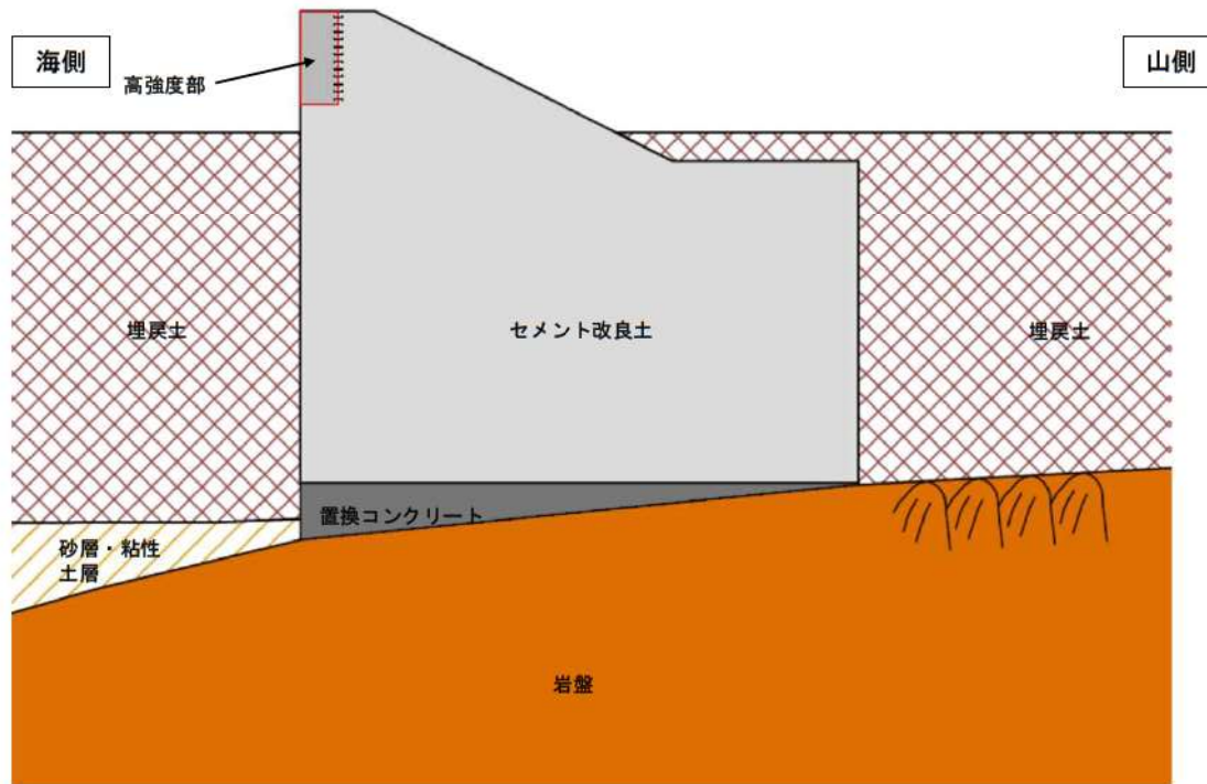
セメント改良土(高強度含む)概要図
