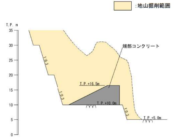
防潮堤掘削側端部断面図
