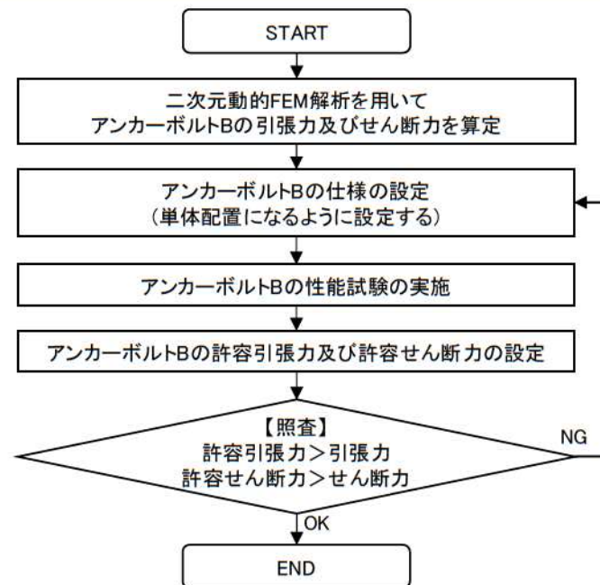
アンカーボルトBの設計フロー
