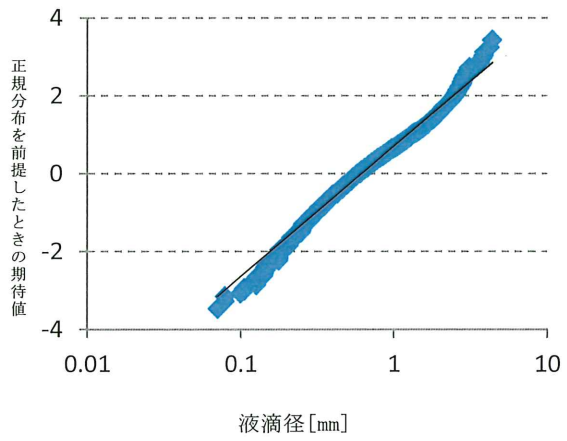
第6-1図 対数正規確率プロット (第1回試験 測定点①～④)
