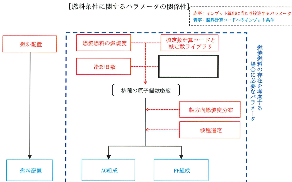
第1-4図 インプット条件とインプット条件算出に当たり設定するパラメータの関係（燃料条件）
