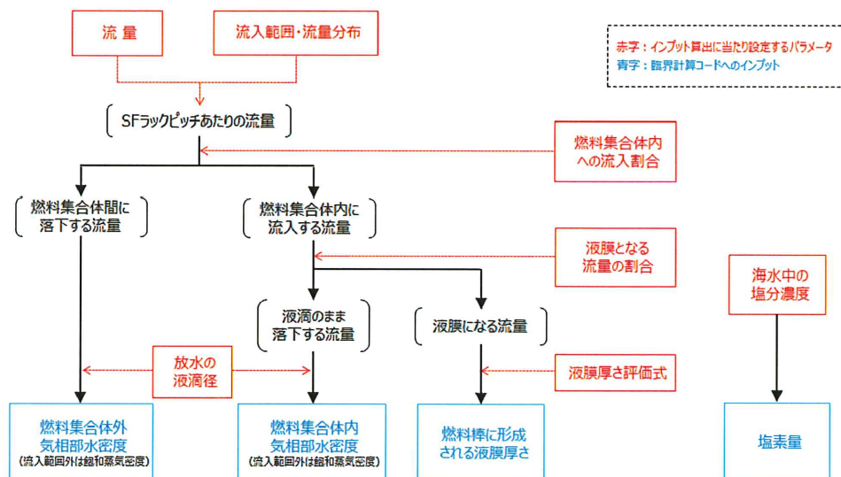
第1-7図 インプット条件とインプット条件算出に当たり設定するパラメータの関係 (水分条件)
