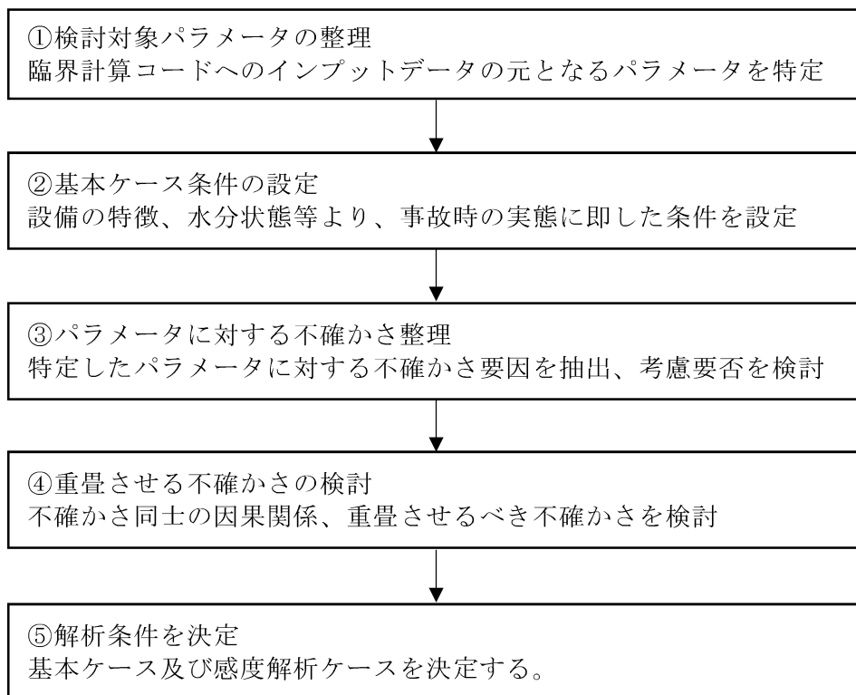
第5図 臨界計算コードの入力データの元となるパラメータの設定フロー
