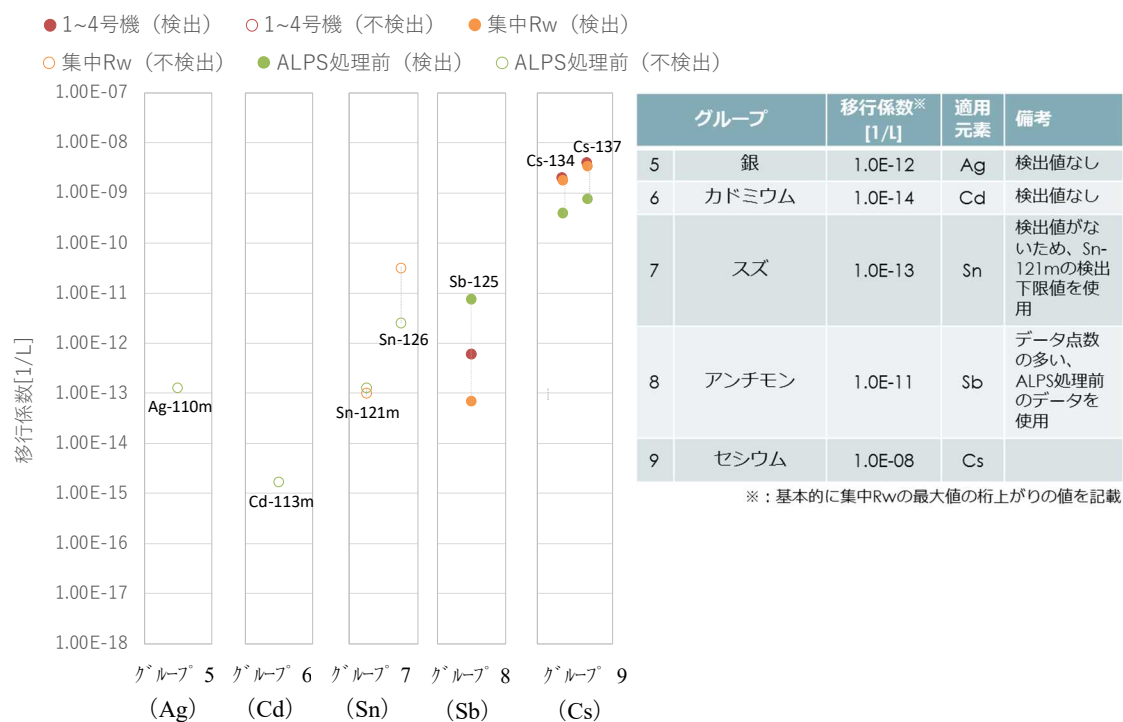
図 1.1.4-9 移行係数 (2/4)
