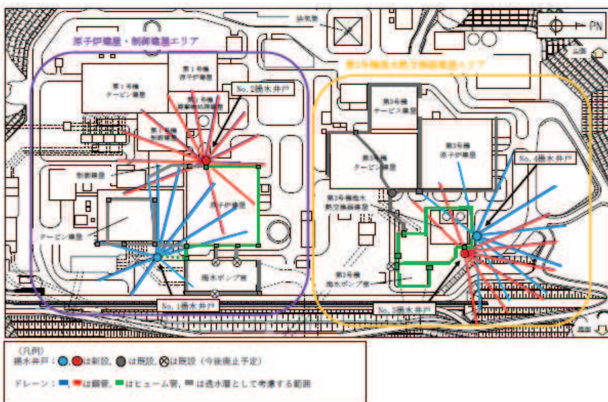
図3-1 地下水位低下設備の配置
