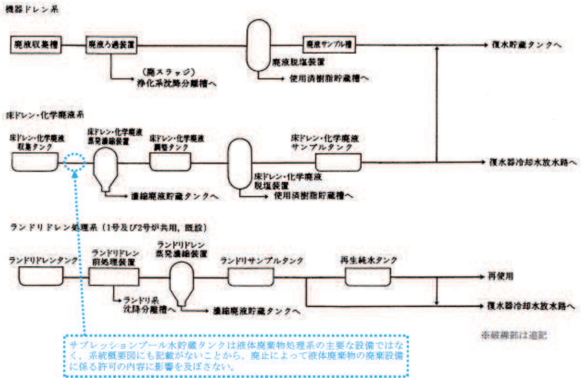
図2 液体廃棄物処理系系統概要図（設置変更許可申請書添付参考図 第21図）
