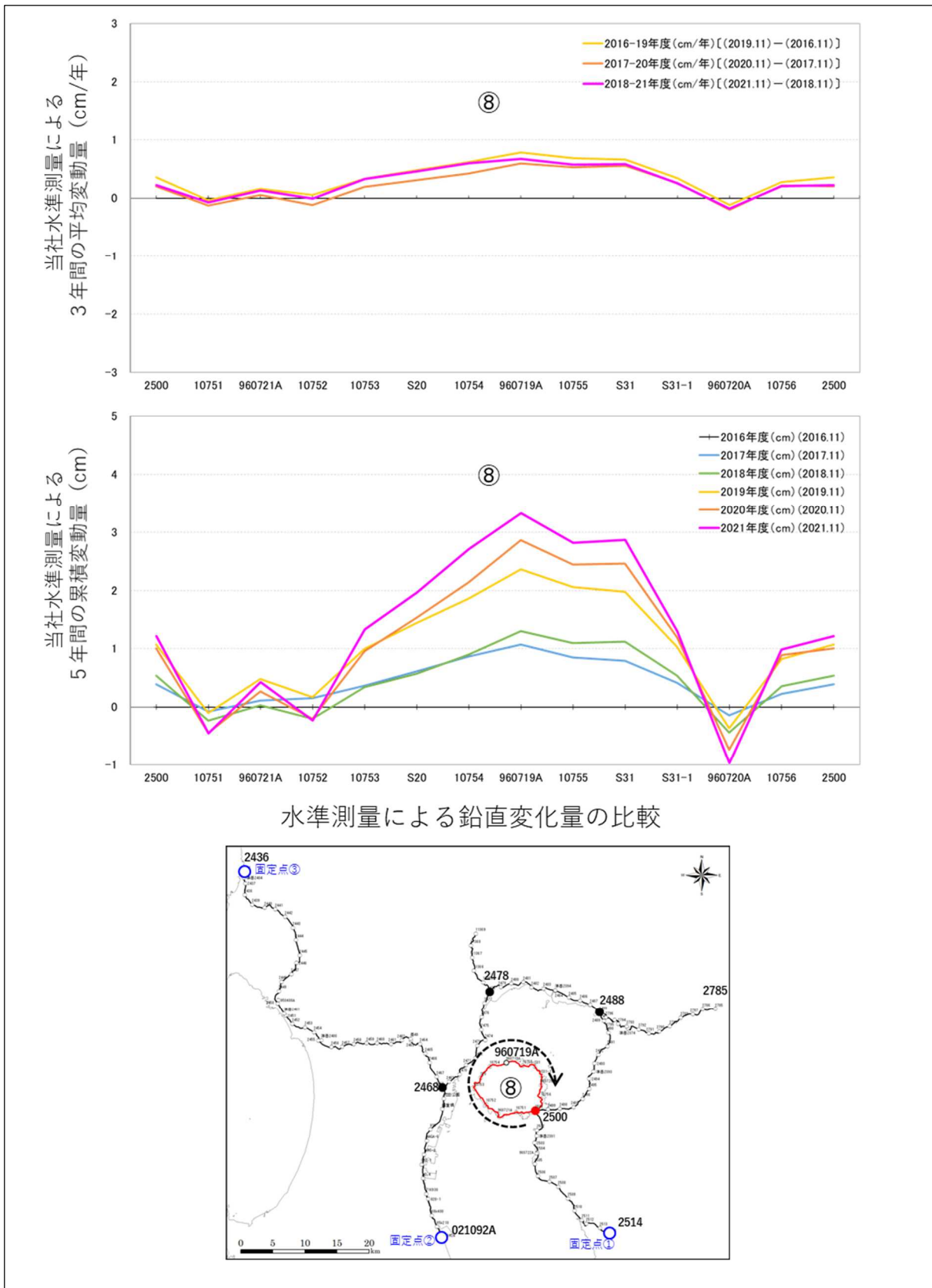
図9 桜島島内の水準測量結果
