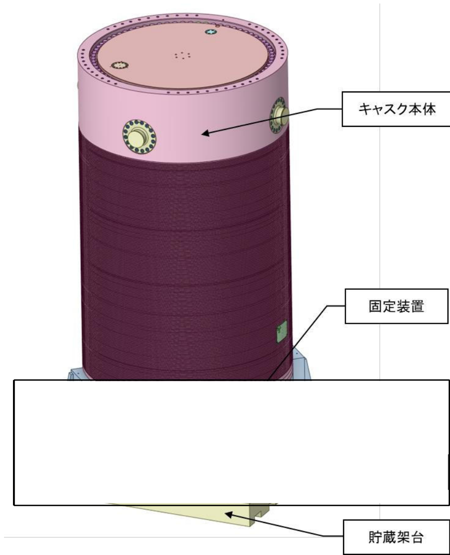
図 A1-1 カセットの固定状態
