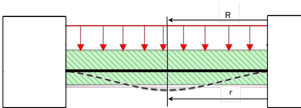
図 A2-2 地震の慣性力に対する一次蓋密封シール部の応力計算モデル
