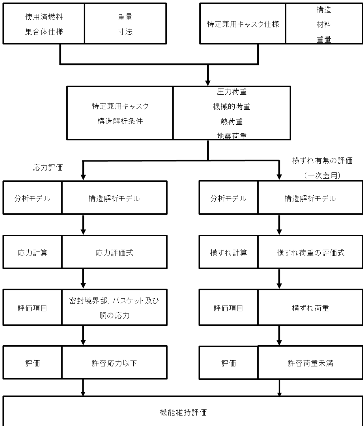
図3 地震時のCASTOR® geo26JP型の機能維持評価フロー
