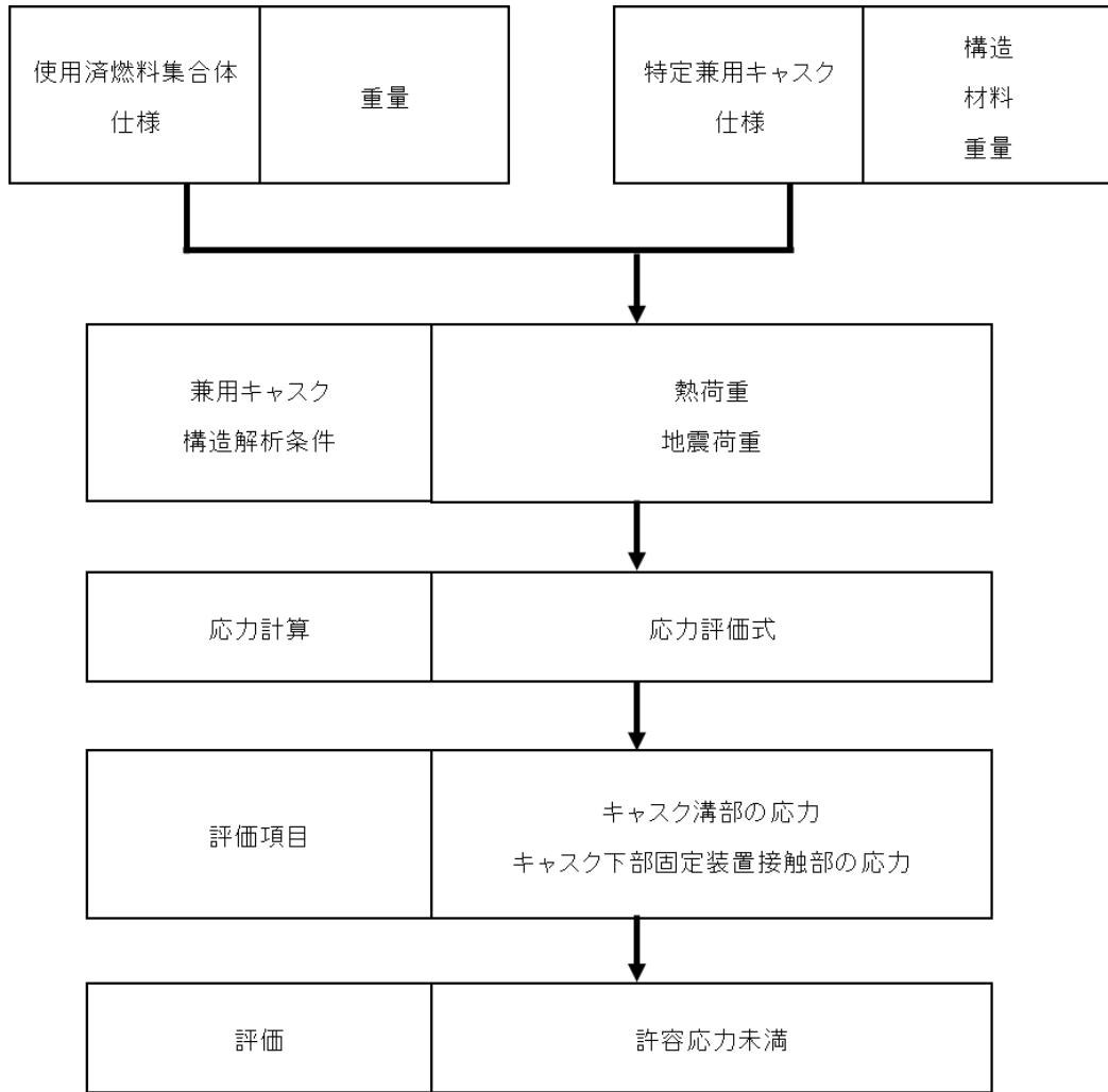
図2 地震時の構造健全性評価フロー
