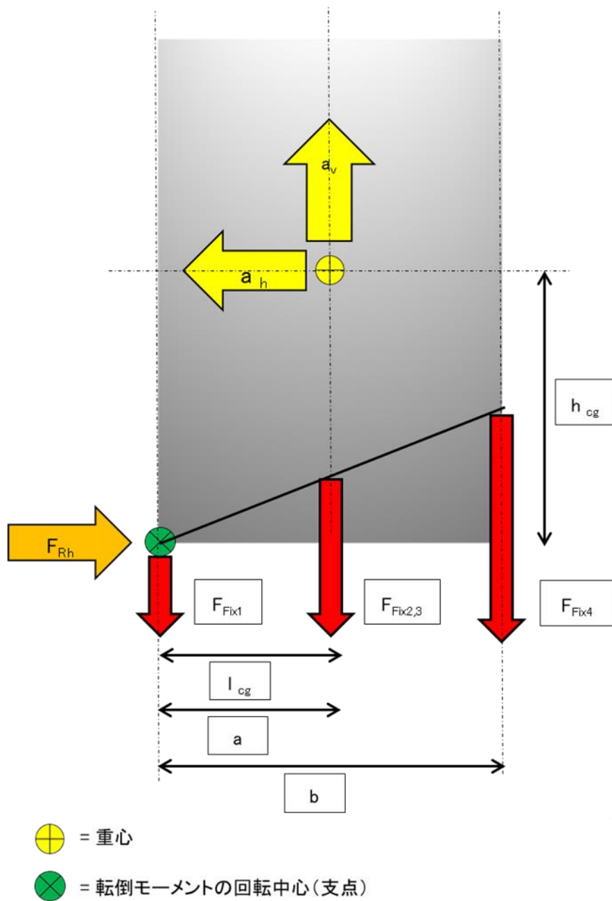
図 A1-5 地震時にキャスク溝部に作用する荷重の概要
