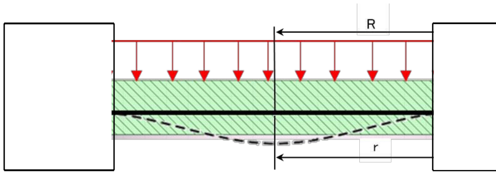
図 A2-1 内圧に対する一次蓋密封シール部の応力計算モデル
