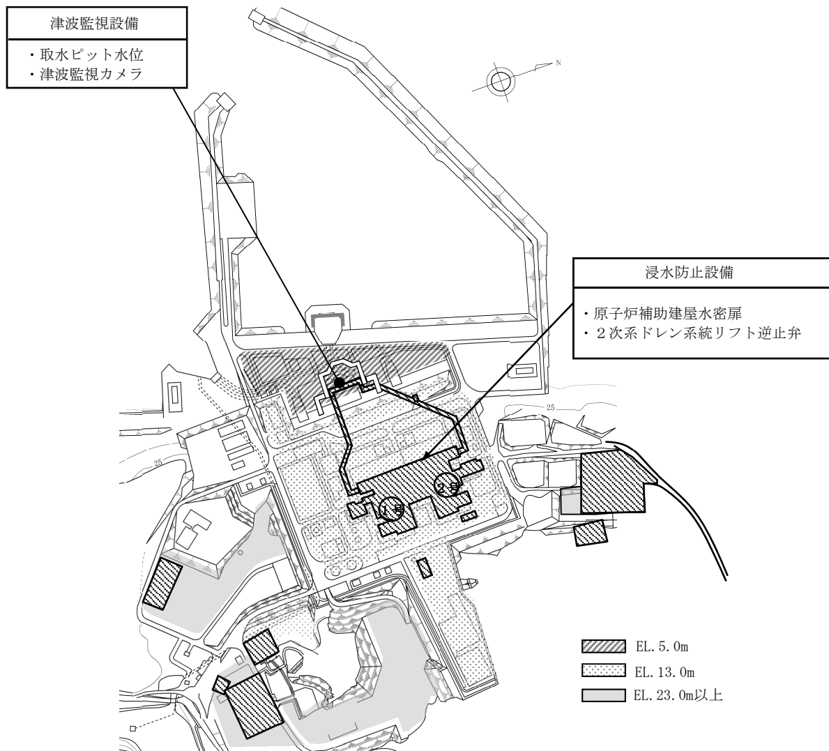
浸水防護施設の概要
