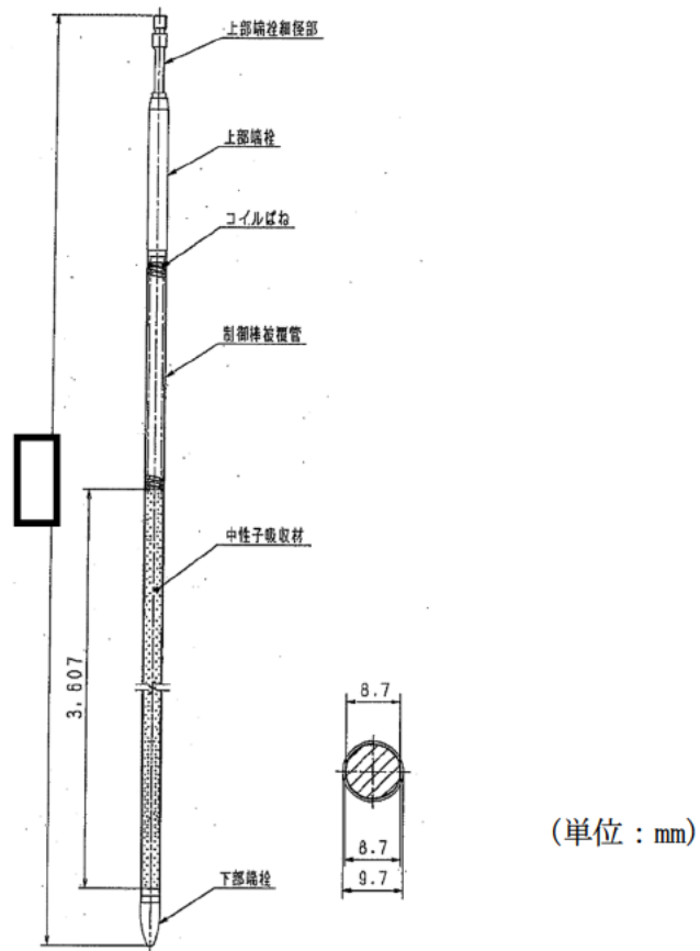
図11-2 17×17型制御棒構造図
