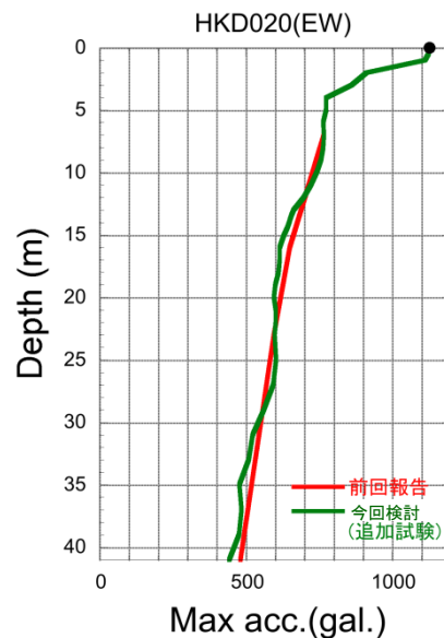
最大加速度
