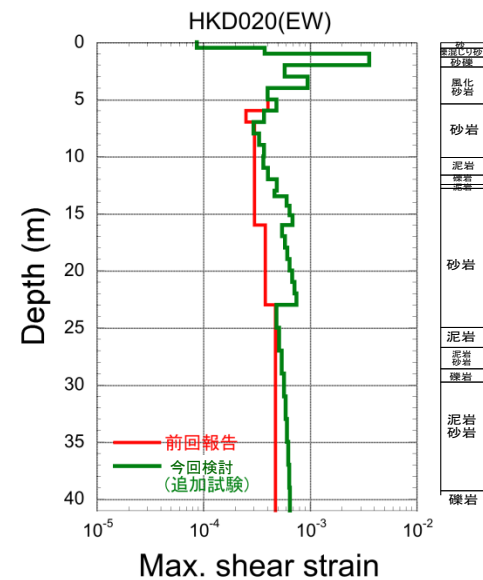
最大ひずみ
