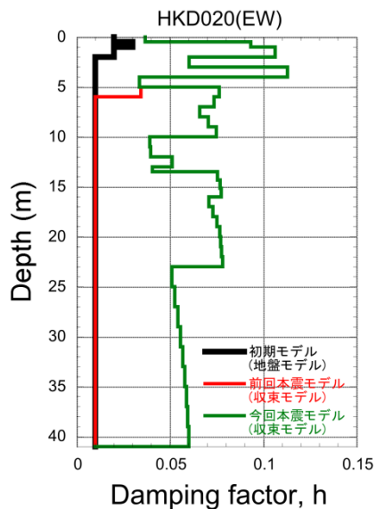
減衰定数
