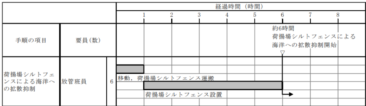
第 1.12.6 図 荷揚場シルトフェンスによる海洋への拡散抑制 タイムチャート
