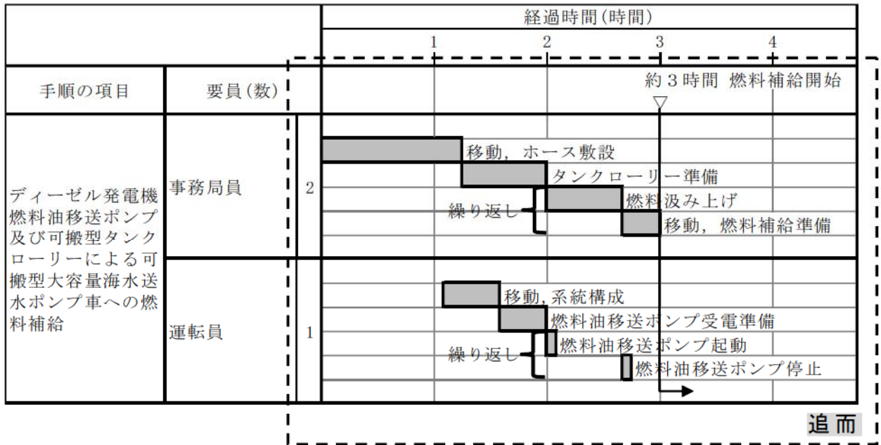
第 1.12.20 図 ディーゼル発電機燃料油移送ポンプ及び可搬型タンクローリーによる可搬型大容量海水送水ポンプ車への燃料補給 タイムチャート
