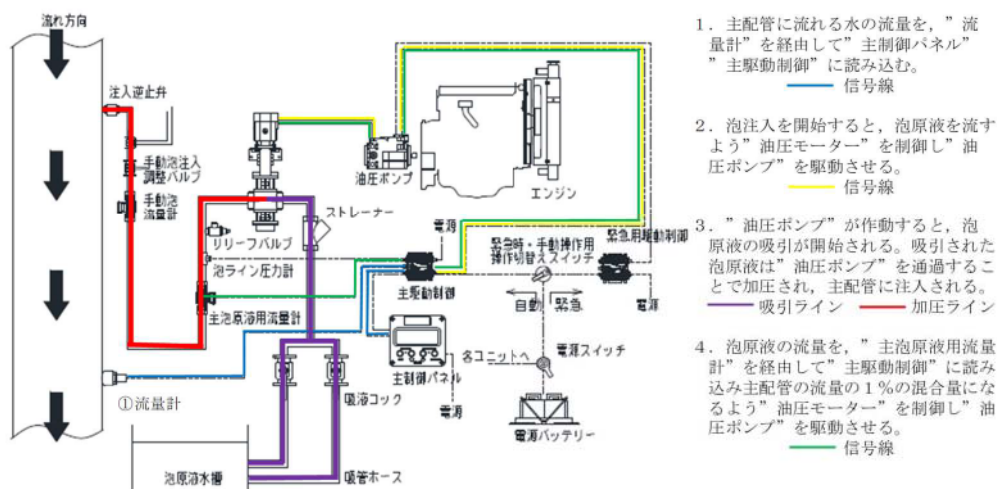
泡混合設備フロー図
