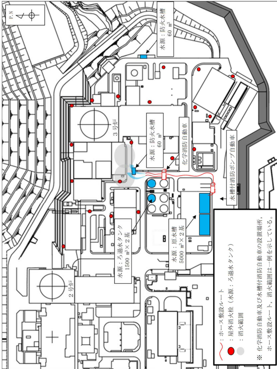
第 1.12.10 図 化学消防自動車及び水タンク付消防ポンプ自動車による泡消火 ホース敷設ルート図
