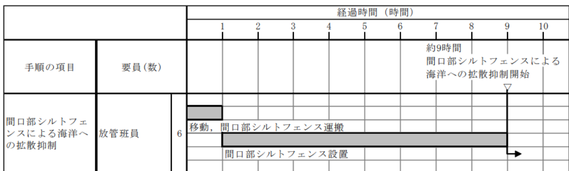
第 1.12.7 図 間口部シルトフェンス海洋への拡散抑制 タイムチャート
