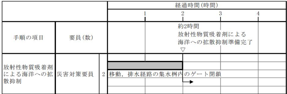
第 1.12.5 図 放射性物質吸着剤による海洋への拡散抑制 タイムチャート
