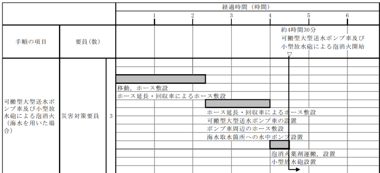
第 1.12.11 図 可搬型大型送水ポンプ車及び小型放水砲による泡消火 タイムチャート
