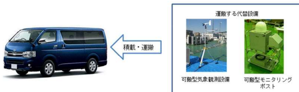
図9 モニタリング資機材運搬車の外観（写真は同型車イメージ）
