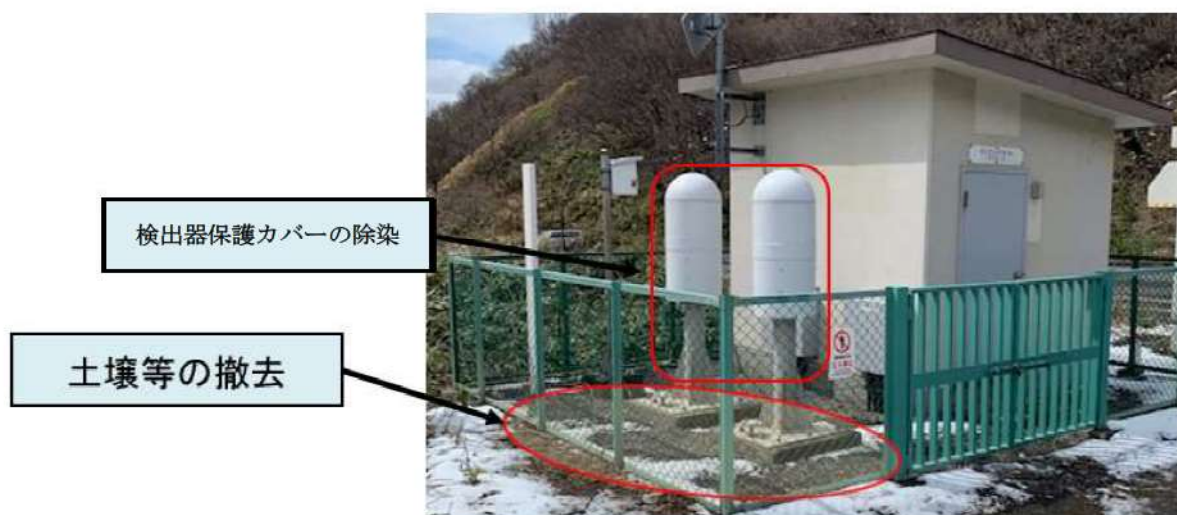
図13 モニタリングポストのバックグラウンド低減対策（イメージ）
